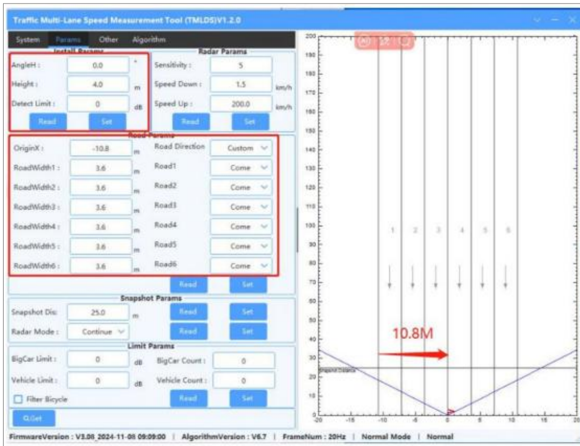
Figura 9 - Configurações de parâmetros para o modo contínuo de aproximação de 0 grau
