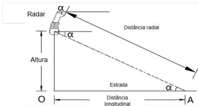
Figura 7 - Diagrama esquemático do radar ajustando o ângulo de inclinação
