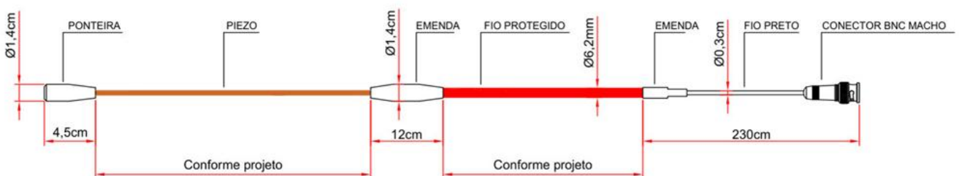
Figura 2 - Sensor de Tráfego ITSENSOR PIEZO
