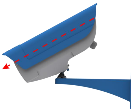
Figura 16 - Ilustração do sentido de prolongamento da cobertura da lente pela Aba Deslizante
