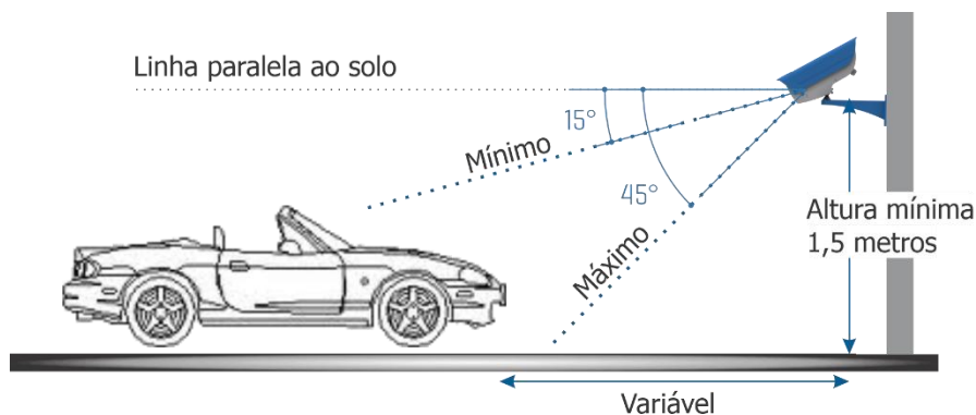
Figura 17 - Vista Lateral da instalação
