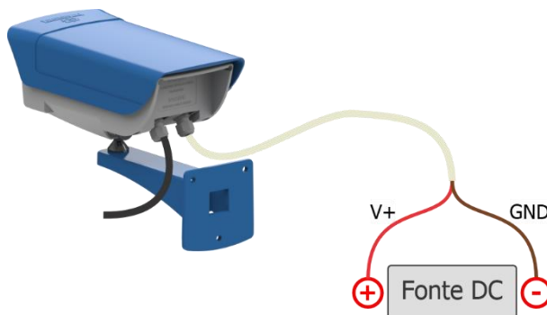
Figura 19 - Conexão de alimentação e sinais da ITSCAM 450+
