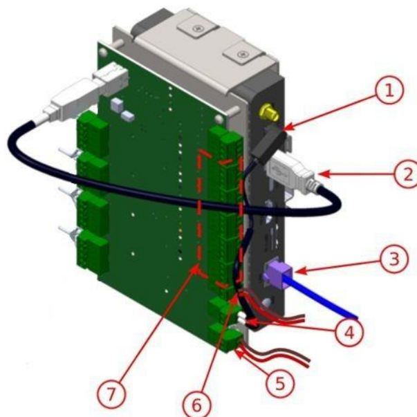
Figura 17 - Conexiones del Módulo Controlador VIGIA-VLIO: 1) Alimentación de la ULP; 2) USB (conexión interna); 3) Ethernet (configuraciones); 4) Alimentación del ULP; 5) Alimentación del Módulo
