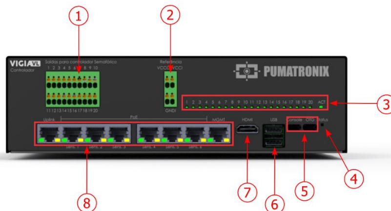
Figura 16 - Interfaces del Nuevo Módulo Controlador VIGIA-VLIO: 1) Salidas para controlador de semáforo; 2) Conexiones para alimentar IOs; 3) LED que indican señales de Salida; 4) LED de estado; 5) entradas microUSB y USB-C; 6) entrada USB; 7) entrada HDMI; 8) Conmutador PoE de 6 puertos
