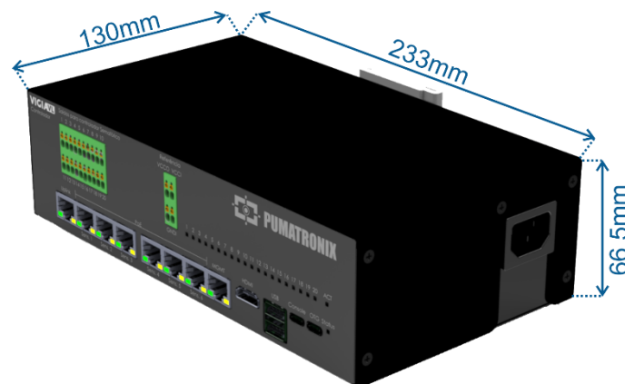
Figura 8 – Dimensiones Nuevo Módulo Controlador
