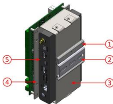
Figura 20 – 1) Soporte carril DIN; 2) Carril DIN 75mm; 3) Soporte inferior; 4) Soporte superior; 5) ULP
