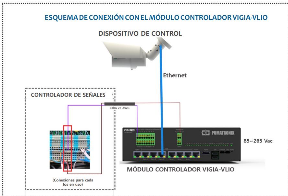
Figura 15 - Esquema de conexión de VIGIA-VL con Nuevo Módulo Controlador
