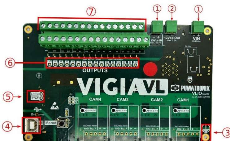
Figura 13 - Interfaces de la placa VLIO: 1) Entradas de alimentación; 2) Conexión de salida para la alimentación de Firefly (ULP); 3) Conexión a tierra de la placa (debe conectarse a la GND de la Instalación); 4) Conexión de datos USB; 5) LEDs de ERROR y STAT; 6) LEDs indicadores de las señales de salida; 7) Salidas de señales hacia el Controlador de Tráfico.
