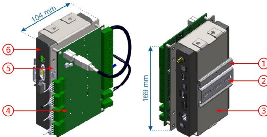
Figura 10 - Módulo Controlador VIGIA-VLIO: 1) Soporte carril DIN; 2) Carril DIN 75mm; 3) Soporte inferior ULP VL; 4) Placa VLIO; 5) Soporte superior ULP VL; 6) ULP
