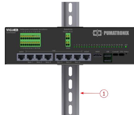
Figura 6 - 1) Carril DIN
