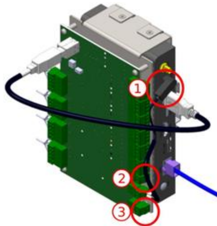
Figura 11 - Conexiones de alimentación en la placa VLIO: 1) Alimentación del módulo controlador VIGIA-VLIO; 2) Alimentación de las E/S aisladas en la placa VLIO; 3) Alimentación de la placa VLIO.
