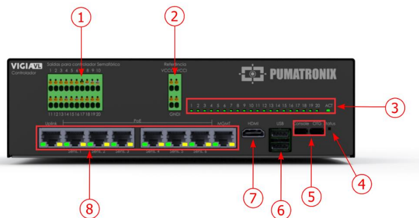
Figura 5 - Interfaces del Nuevo Módulo Controlador VIGIA-VLIO: 1) Salidas para controlador de semáforo; 2) Salidas Vcc-Out, Vcc-In y GND; 3) LED que indican señales de Salida; 4) LED de estado; 5) entradas microUSB y USB-C; 6) entrada USB; 7) entrada HDMI; 8) Conmutador PoE de 6 puertos
