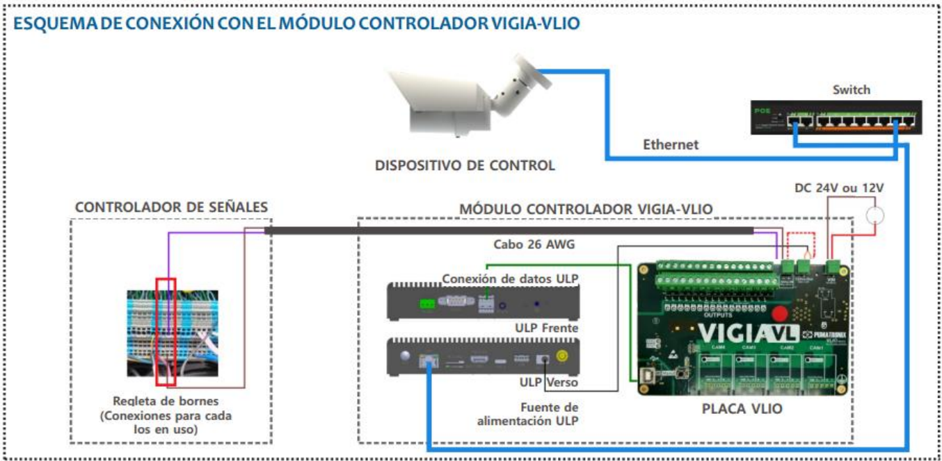
Figura 14 - Esquema de conexión de VIGIA-VL
