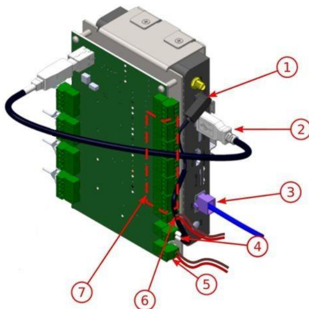
Figura 17 - Conexiones del Módulo Controlador VIGIA-VLIO: 1) Alimentación de la ULP; 2) USB (conexión interna); 3) Ethernet (configuraciones); 4) Alimentación del ULP; 5) Alimentación del Módulo Controlador VIGIA-VLIO; 6) Alimentación de las salidas aisladas; 7) Salidas (conexión con el Controlador de Semáforos)
