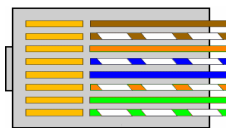
Figura 13 - Conector RJ-45 estándar EIA/TIA-568A
