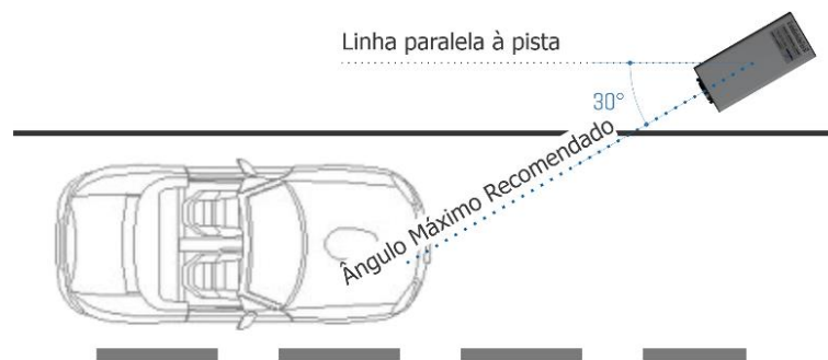
Figura 19 - Vista Superior da instalação
