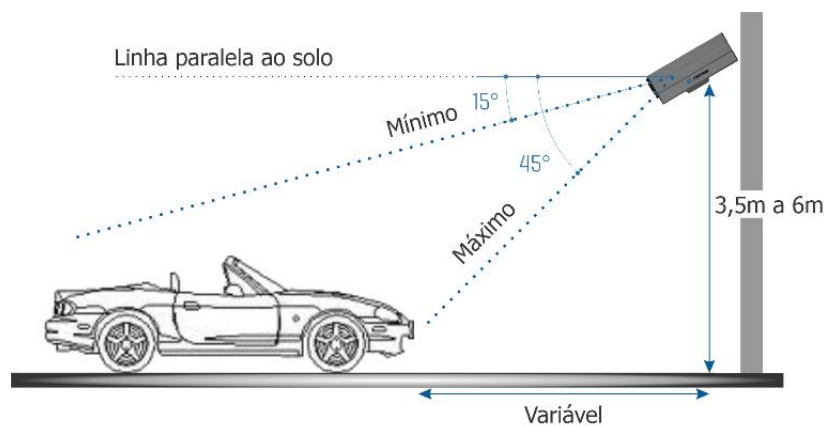
Figura 18 - Vista Lateral da instalação
