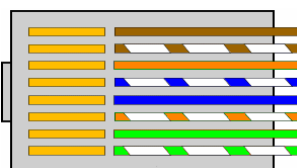
Figura 8 - Conector RJ-45 padrão EIA/TIA-568A
