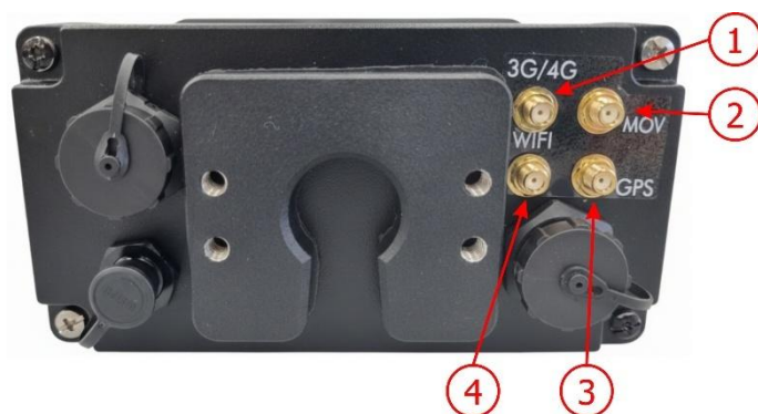
Figura 9 – Pontos de conexão das antenas* na VTR 600
