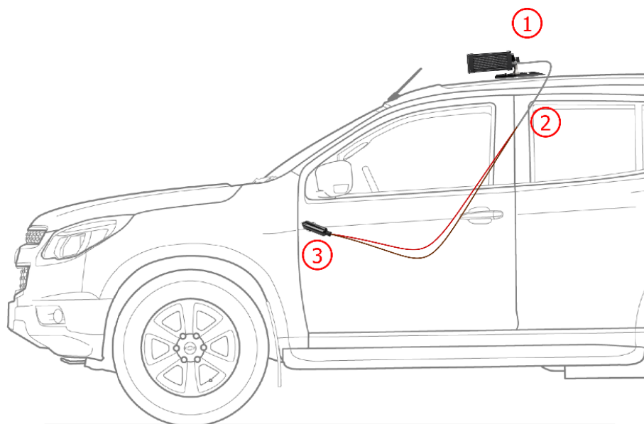
Figura 7 - Modelo de instalação utilizando o acendedor de cigarros na alimentação: 1) VTR 600 fixo ao teto do veículo, 2) Cabo manga 2 vias 12Vdc, 3) Plug conectado ao acendedor de cigarros veicular
