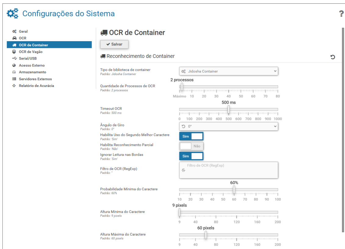
Figura 23 - Tela em Configurações de Sistema > OCR de Container
