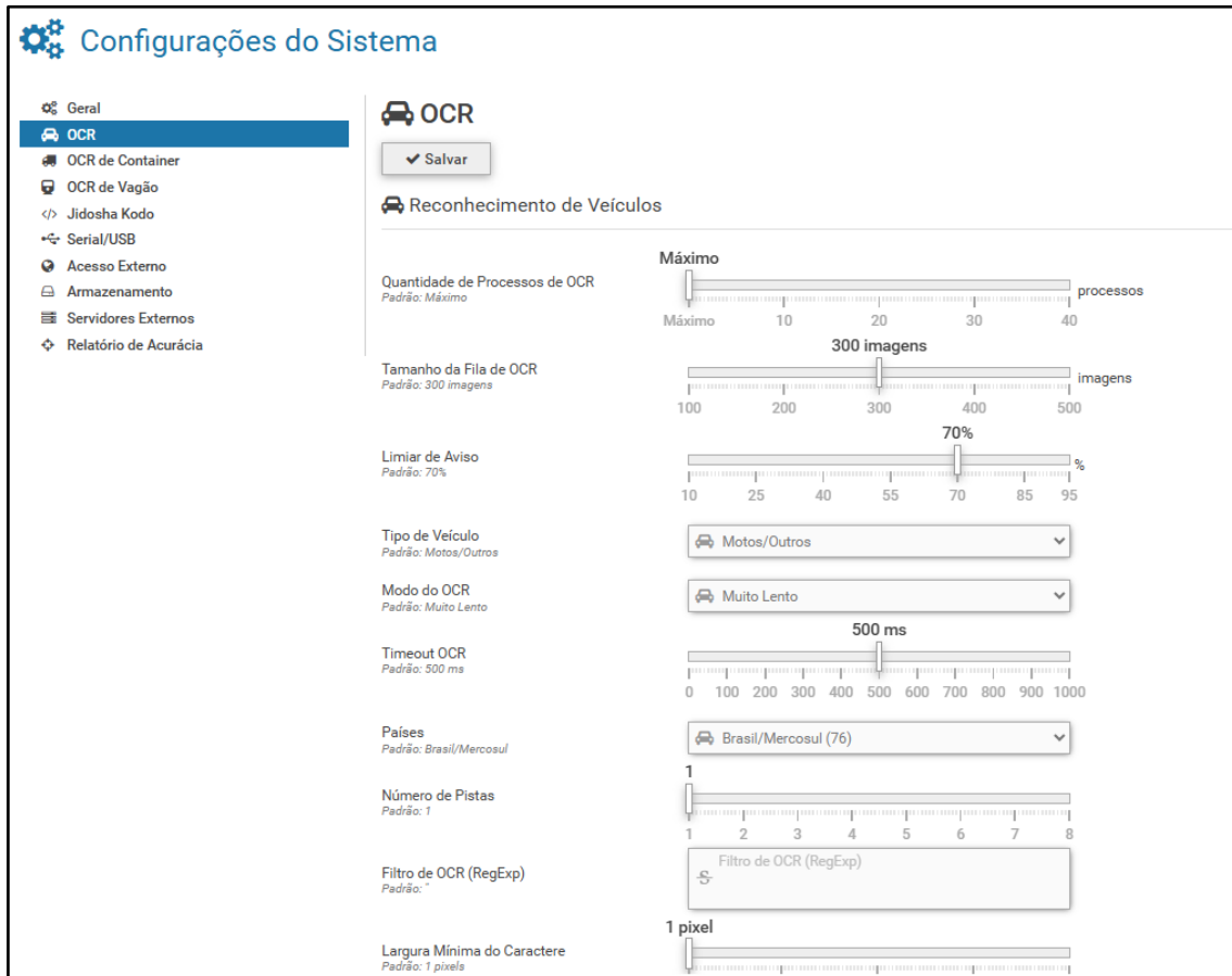
Figura 22 – Tela em Configurações do Sistema > OCR
