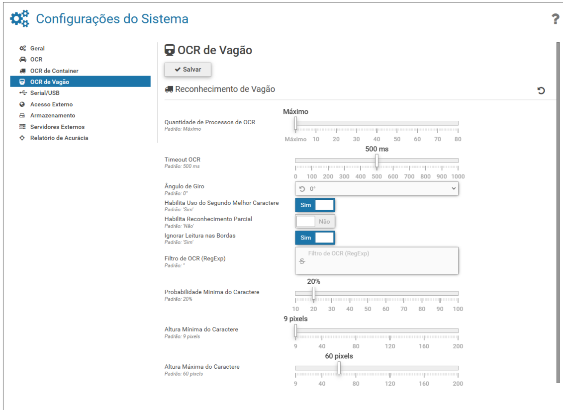
Figura 24 - Tela em Configurações de Sistema > OCR de Vagão
