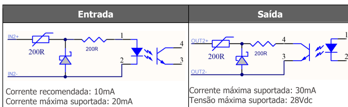
Figura 36 - Circuito dos sinais de entrada/ saída isoladas da ITSCAM 400
