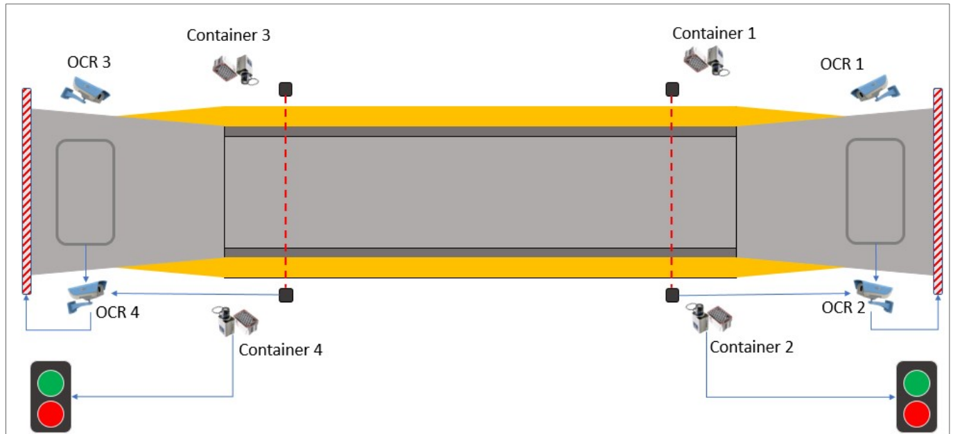
Figura 14 – Diagrama da Arquitetura do Sistema WeGate
