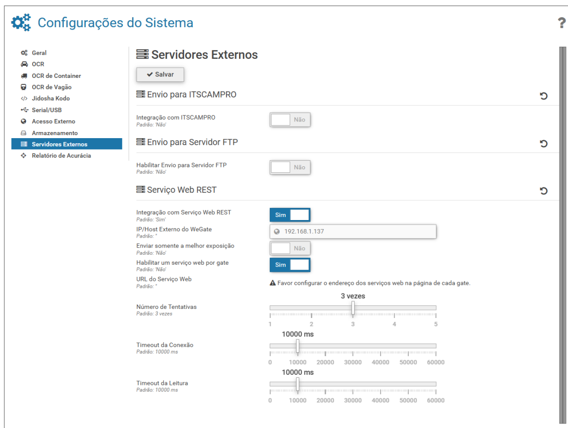
Figura 28 – Tela em Configurações do Sistema > Servidores Externos > Serviço Web REST
