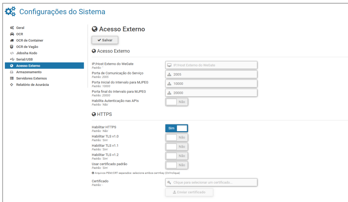
Figura 29 - Tela em Configurações do Sistema > Acesso Externo
