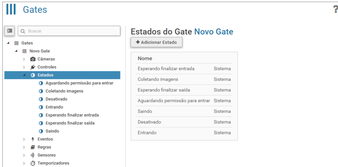
Figura 41 - Tela em Gates > Novo Gate > Estados
