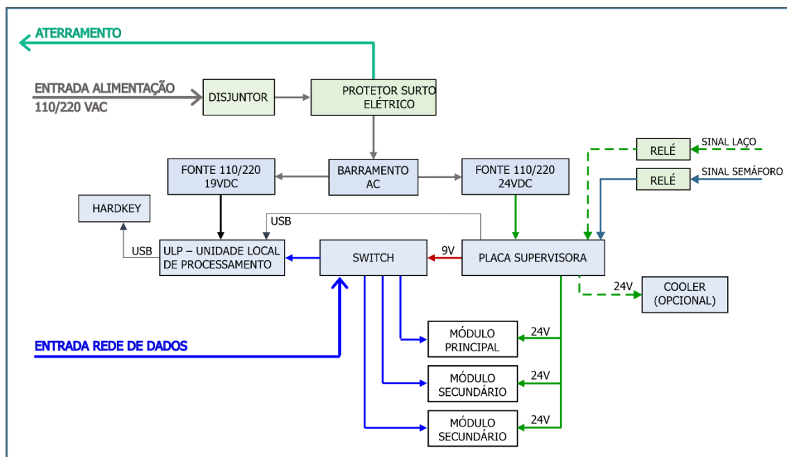
Figura 17 - Diagrama Elétrico* das Conexões no Módulo Terciário com Quadro NM1
