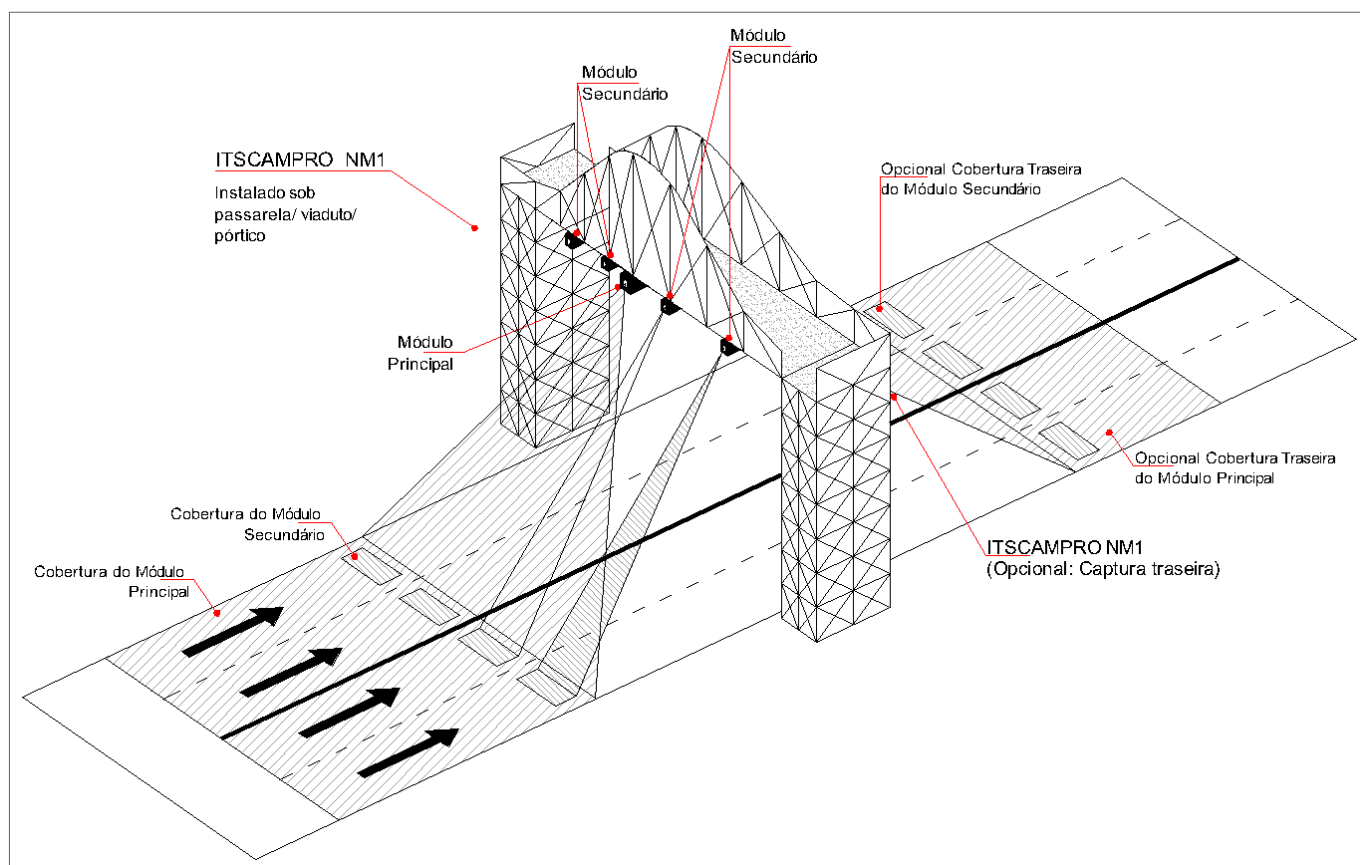
Figura 27 - Exemplos de fixação em Pórticos
