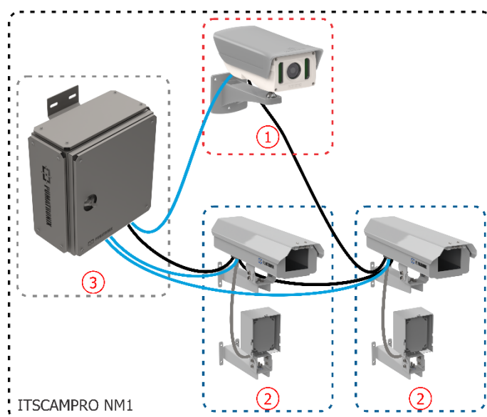
Figura 2 - Diagrama ilustrativo da conexão entre os Módulos do ITSCAMPRO NM1: 1) Módulo Principal, 2) Módulo Secundário, 3) Módulo Terciário
