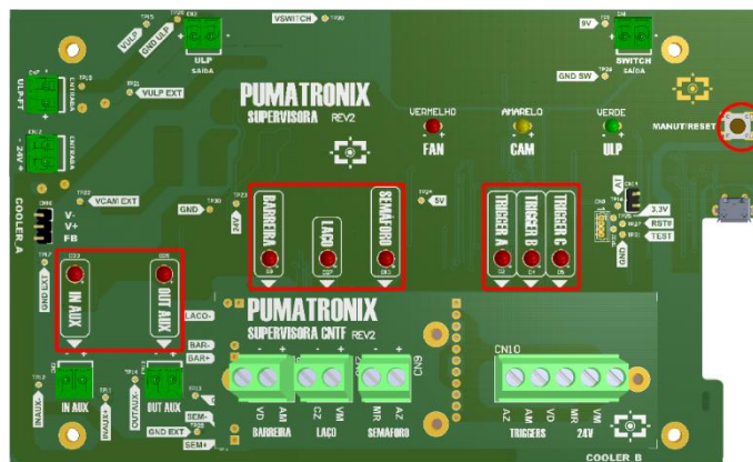
Figura 20 - Posição dos LEDs na Placa Supervisora Rev2
