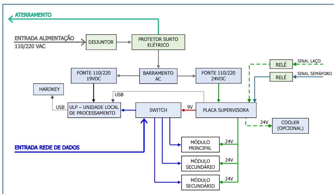
Figura 18 - Diagrama Elétrico* das Conexões no Módulo Terciário com Quadro NM1 Compacto
