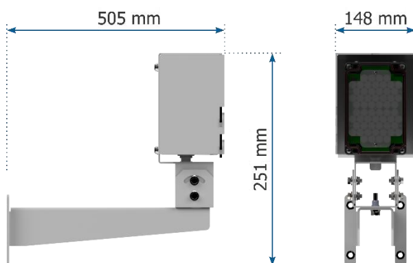
Figura 11 - ITSLUX com suporte
