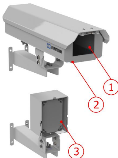
Figura 8 - Módulo Secundário: 1) ITSCAM 411, 2) Caixa de Proteção PTX12, 3) ITSLUX com suporte
