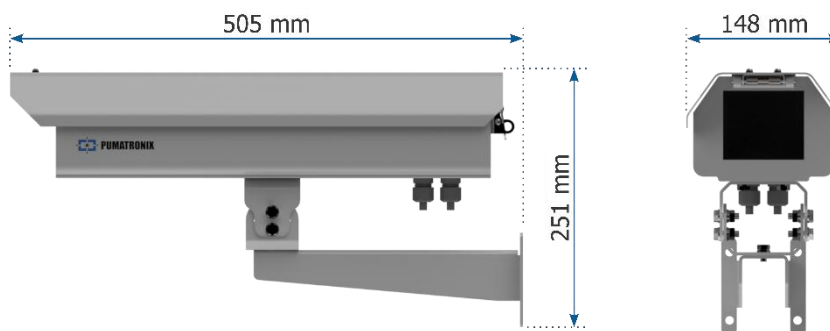
Figura 9 - Dimensões da Caixa de Proteção PTX12
