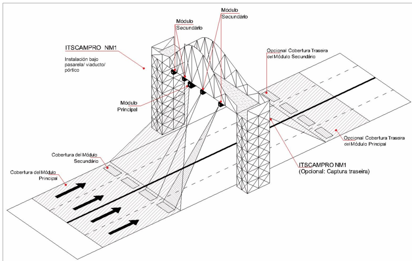
Figura 27- Ejemplos de fijación en Pórticos
