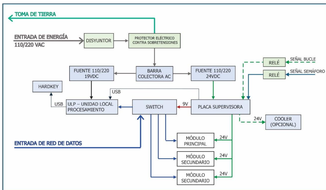
Figura17- Diagrama Eléctrico* de Conexiones en Módulo Terciario con Cuadro NM1
