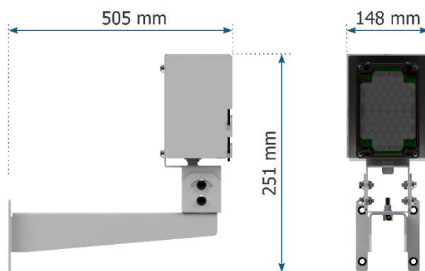
Figura11 - ITSLUX con soporte
