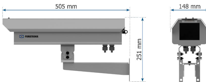
Figura 9 - Dimensiones de la caja de protección PTX12
