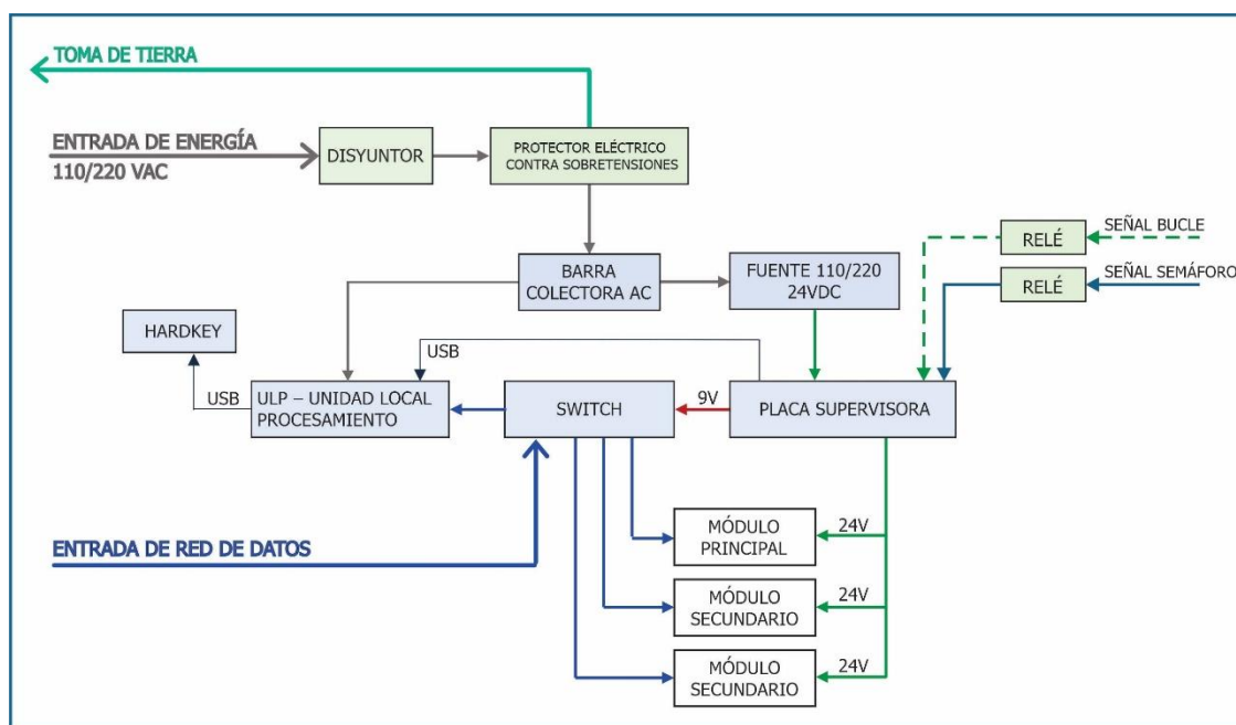
Figura 18 - Diagrama Eléctrico* de Conexiones en Módulo Terciario con Cuadro NM1 Compacto
