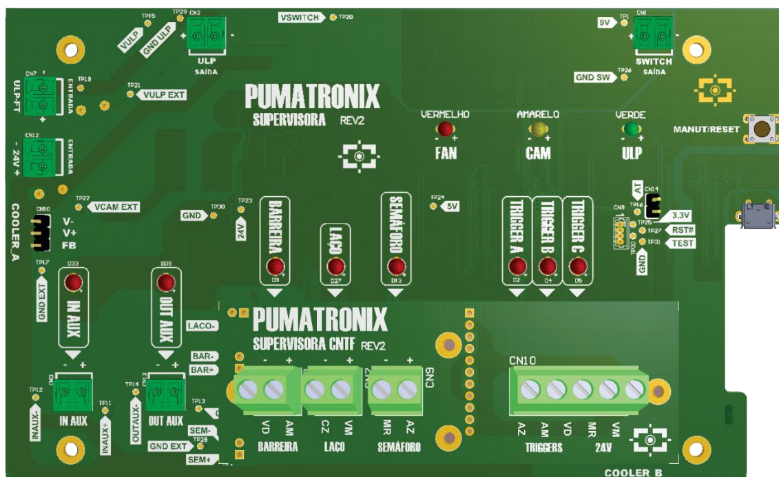
Figura 19 - Placa Supervisora Rev2
