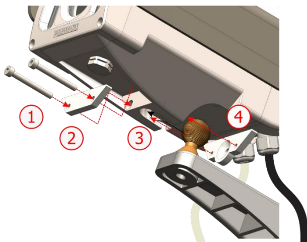
Figura 7 - Montaje del WATCHMAN+ Sujetador: 1) Tornillos Allen M4 3mm (2 unidades); 2) Refuerzo; 3) WATCHMAN+ cavidad; 4) Sujetador
