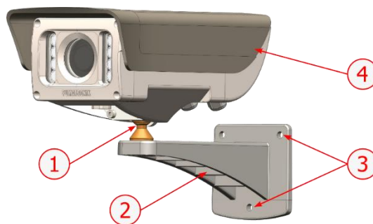
Figura 6 - Fijación del Soporte VIGIA+: 1) Ajuste de inclinación del dispositivo VIGIA+; 2) Soporte VIGIA+; 3) Puntos de fijación, utilizando tornillos de 3/16"; 4) Solapa deslizante, ajustada en el encuadre
