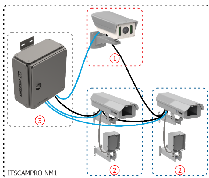
Figura 2 - Diagrama ilustrativo de la conexión entre los Módulos ITSCAMPRO NM1: 1) Módulo Principal, 2) Módulo Secundario, 3) Módulo Terciario
