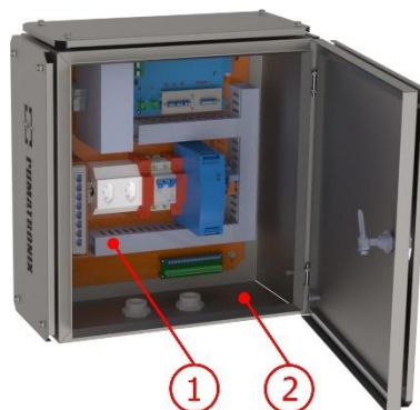
Figura 14- Módulo Terciario con Cuadro NM1 Compacto: 1) Dispositivos eléctricos; 2) Cuadro NM1
