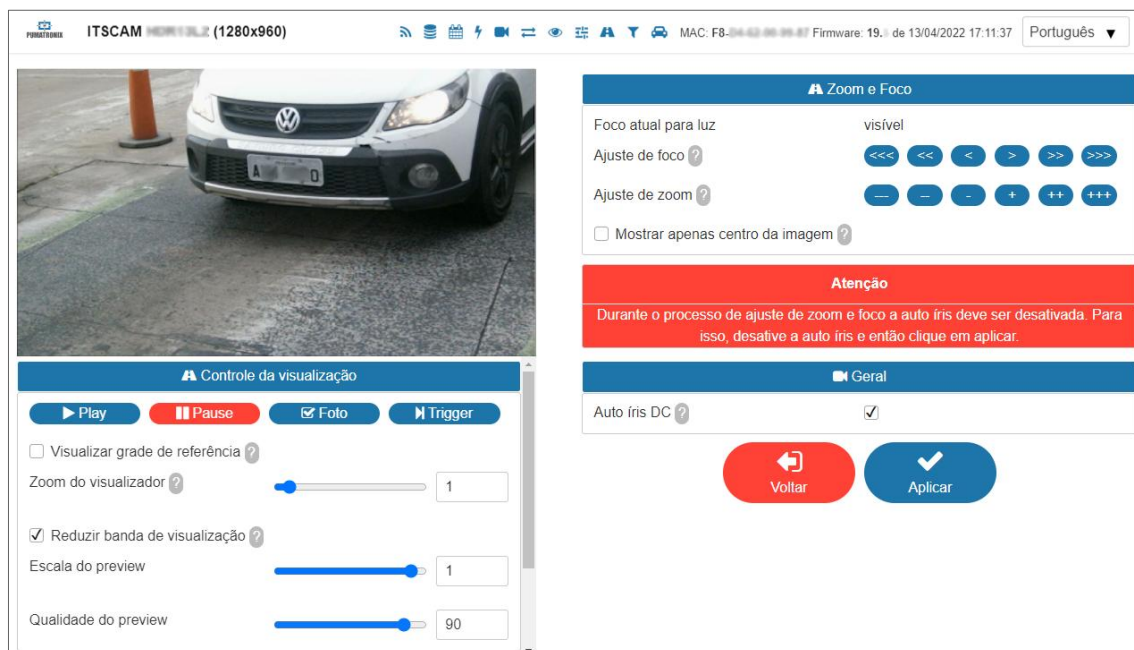
Figura 29 – Ejemplo de pantalla de la interfaz web del dispositivo ITSCAM con la vista previa de la imagen y las opciones de zoom y enfoque
