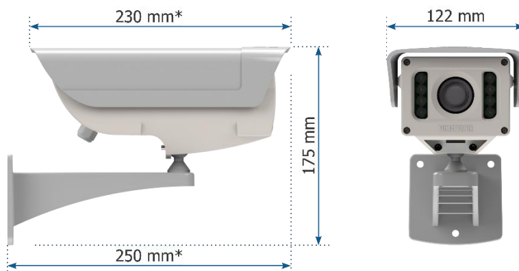
Figura 5 - Dimensiones de ITSCAM VIGIA+
