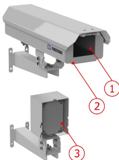
Figura 8 - Módulo Secundario: 1) ITSCAM 411, 2) Caja de Protección PTX12, 3) ITSLUX con soporte
