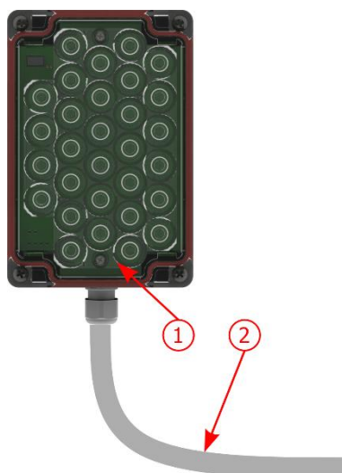
Figura 12 - Interfaz ITSLUX: 1) LED indicativo de funcionamiento; 2) Cable de manga de 6 vías
