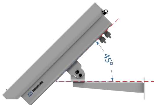
Figura 19 - Ângulo máximo de inclinação da Caixa de Proteção da ITSCAM FF 600
