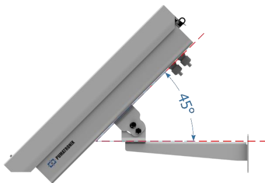
Figura 19 - Ângulo máximo de inclinação da Caixa de Proteção da ITSCAM FF 600
