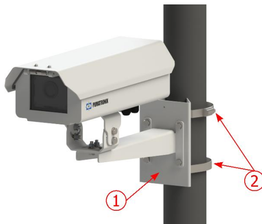
Figura 8 - Fixação em poste: 1) Suporte para Poste; 2) Abraçadeira em inox
