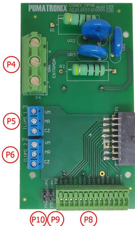
Figura 11 - Placa de Conexões do modelo ITSCAM FF 450 (CP6I7)
