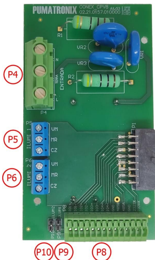
Figura 11 - Placa de conexión para el modelo ITSCAM FF 450 (CP117)
