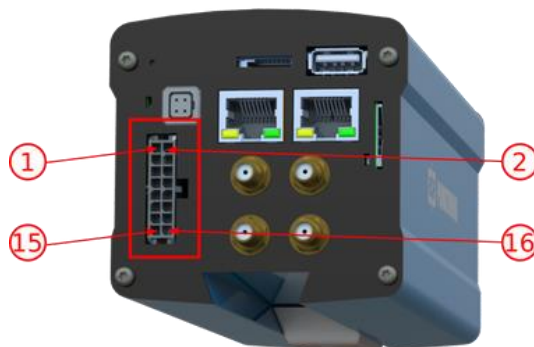
Figura 24 - Conector de alimentação e sinais (Microfit) da ITSCAM 600
