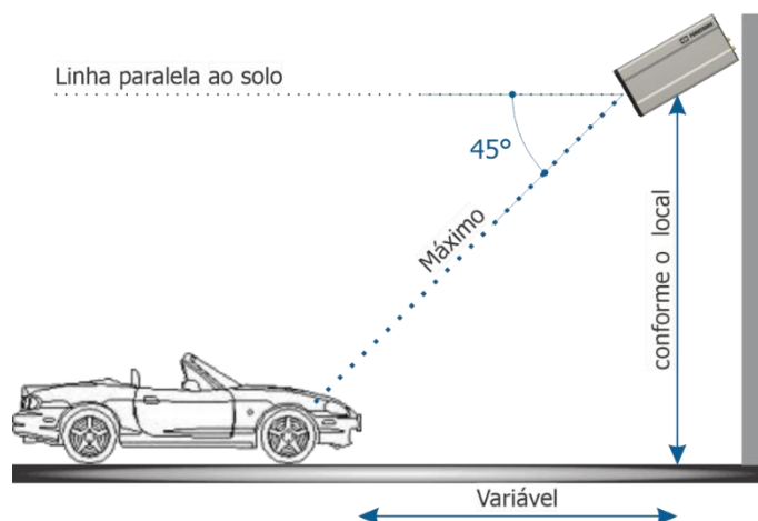
Figura 23 - Vista Lateral da instalação
