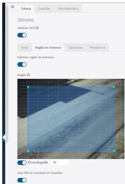
Figura 21 – Interface Web para configuração da ROI (Região de Interesse) do OCR
