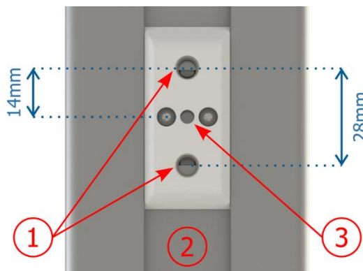
Figura 11 - Especificações do Mecanismo de Fixação: 1) Rosca para parafusos \frac{1}{4} \";
