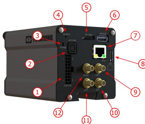
Figura 13 - Interfaces de la línea ITSCAM 600 (puede haber variaciones según el modelo)
