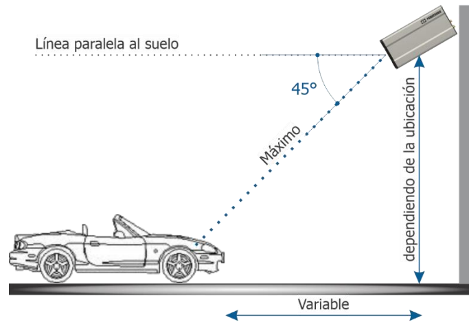
Figura 24 - Vista lateral de la instalación
