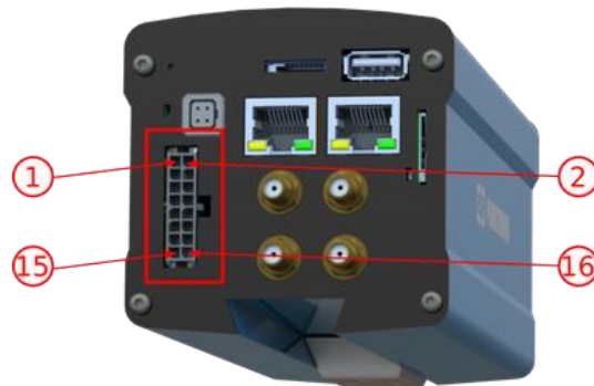
Figura 25 – Conector de alimentación y señales (Microfit) de la ITSCAM 600
