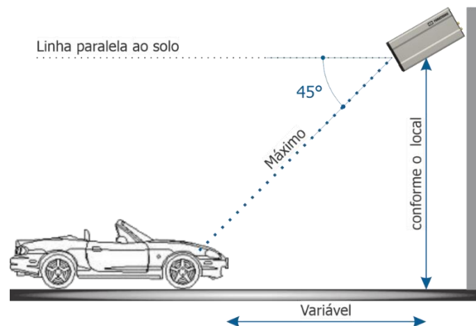
Figura 24 - Vista Lateral da instalação
