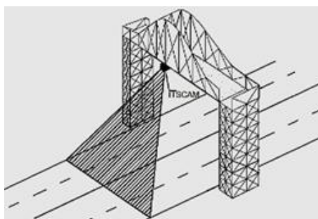
Figura 5 - Instalación de ITSCAM 400 para maximizar los resultados del uso de la función de Contador de Vehículos
