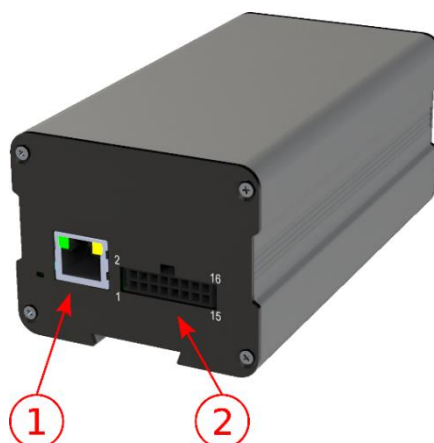
Figura 9 – Interfaces disponíveis no dispositivo: 1) Ethernet; 2) Microfit 16 vias (conector alimentação, IOs, RS-232)
