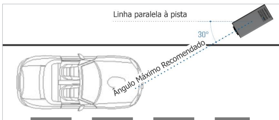
Figura 18 - Vista Superior da instalação
