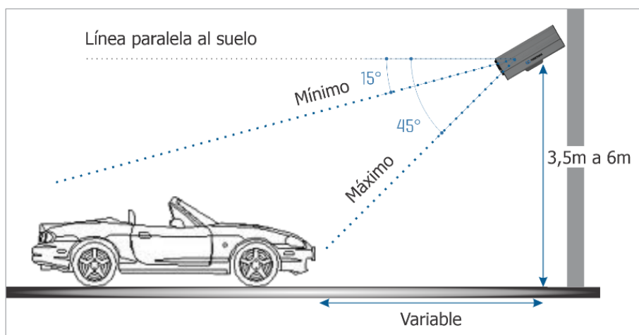
Figura 17 - Vista lateral de la instalación Posicionamiento Frontal
