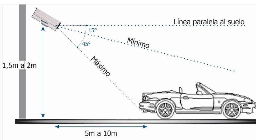
Figure 19 - Vista lateral de la instalación Posicionamiento Trasero
