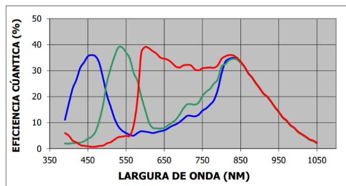
Figura 10 - Sensibilidad roja, verde y azul en el sensor en color
