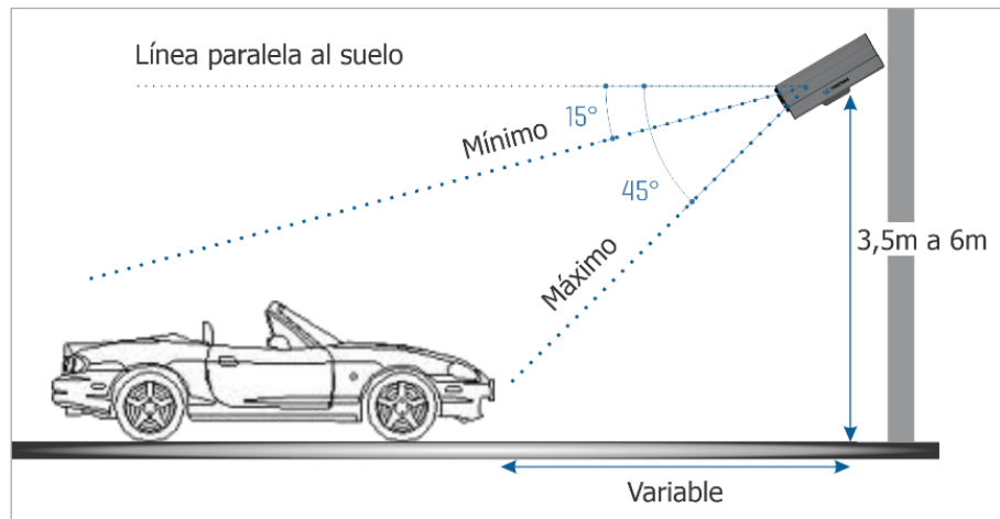
Figura 17 - Vista lateral de la instalación
