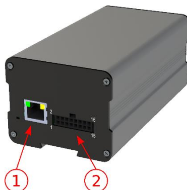
Figura 9 - Interfaces disponibles en el dispositivo: 1) Ethernet; 2) Microfit de 16 vías (conector de alimentación, E/S, RS-232)
