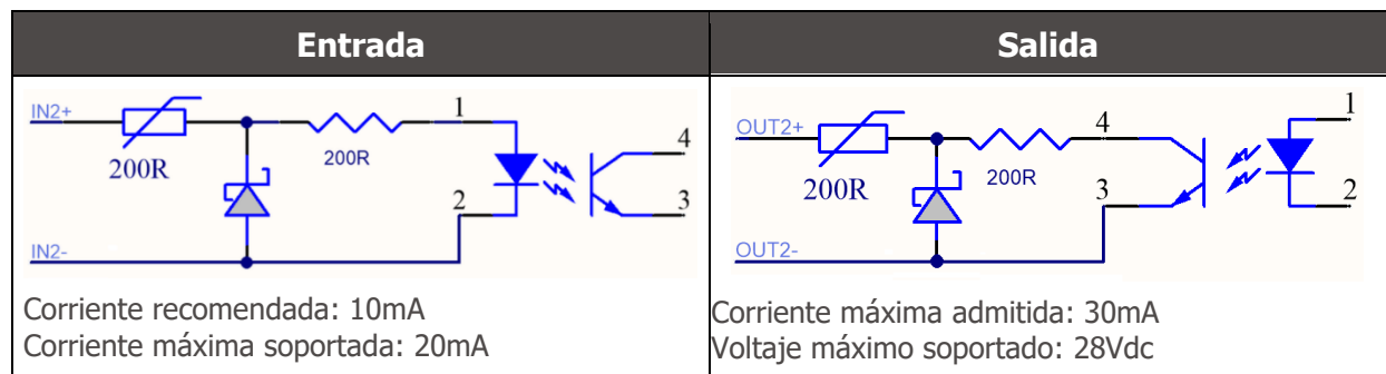
Figura 12 - Circuito de las señales aisladas de entrada/salida de la ITSCAM 400
