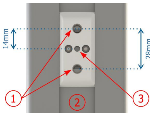
Figura 7 - Especificaciones del Mecanismo de Fijación: 1) Rosca de tornillo 1/4"; 2) Carril para cambiar el punto de fijación; 3) Orificio Ø4mm para el pasador guía
