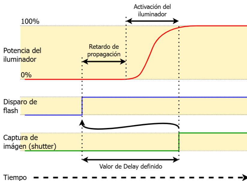
Figura 13 - Momento de accionamiento del obturador (shutter) después de la intensificación del flash
