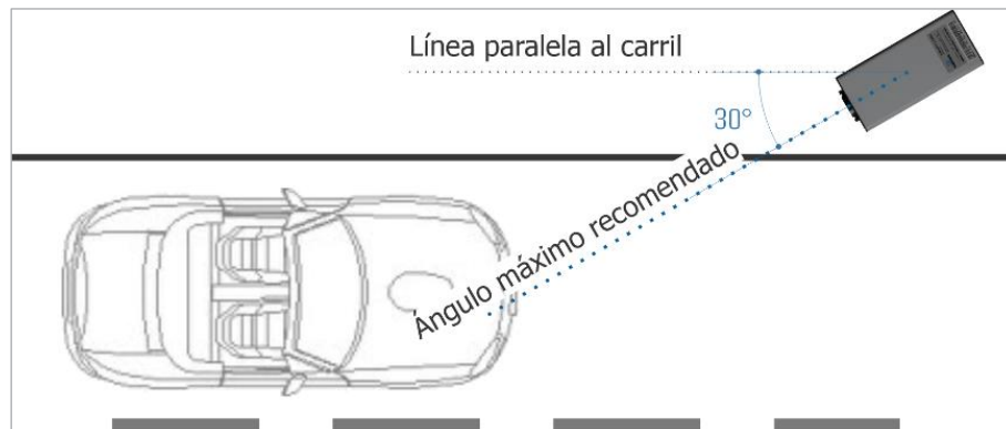
Figura 18 - Vista superior de la instalación
