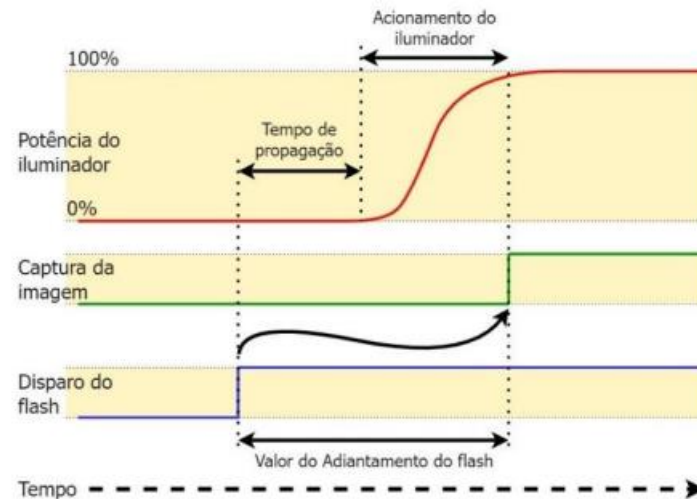
Figura 13 - Momento de accionamiento del obturador (shutter) después de la intensificación del flash
