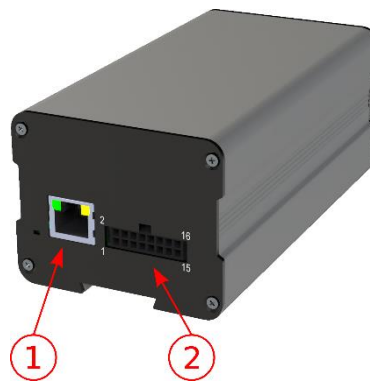
Figura 9 - Interfaces disponibles en el dispositivo: 1) Ethernet; 2) Microfit de 16 vías (conector de alimentación, E/S, RS-232)
