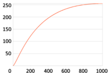
Figura 21 - Ejemplo de la curva de Gamma 140, que convierte de forma logarítmica los valores de cada píxel de la imagen
