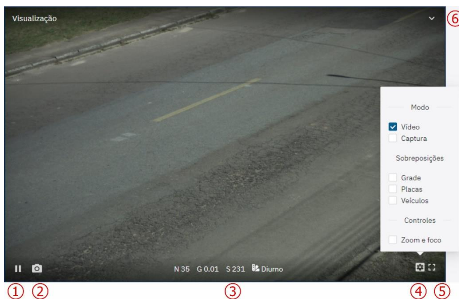
Figura 18 – Janela flutuante de visualização ao vivo: 1) Pausar visualização ao vivo; 2) Tirar foto; 3) Valores de Nível , Ganho , Shutter e Perfil de Imagem ativos; 4) Configurações de visualização; 5) Tela inteira; 6) Minimizar janela
