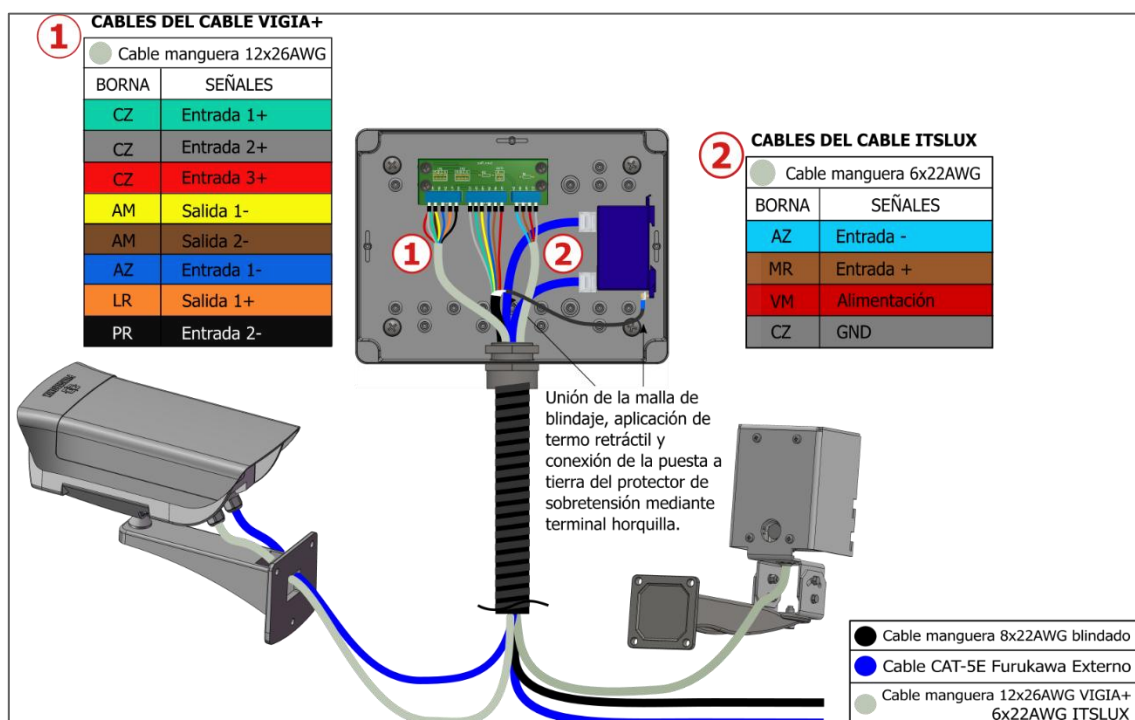
Figura 19 - Diagrama de Conexiones del dispositivo ITSCAM VIGIA+ e ITSLUX en el Poste Frontal con placa de conexión 1.0
