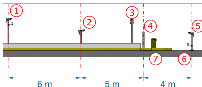
Figura 2 - Vista lateral de la instalación en una pista de cobro automático (AVI): 1) Poste de captura Panorámica, 2) Poste de captura Trasera, 3) Semáforo de la pista, 4) Barrera Óptica de la pista, 5) Poste de captura Frontal, 6) Lazo de la pista, 7) Barrera de la pista
