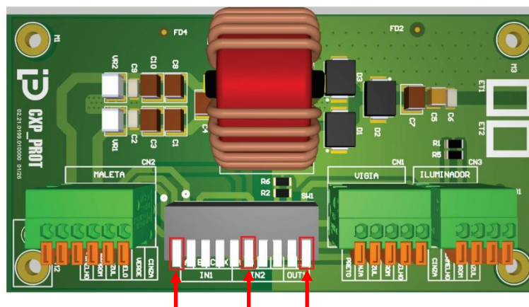
Figura 30 – Ejemplo de configuración de la placa de conexión 2.0 de la Caja de Paso para el dispositivo de captura de imagen Frontal
