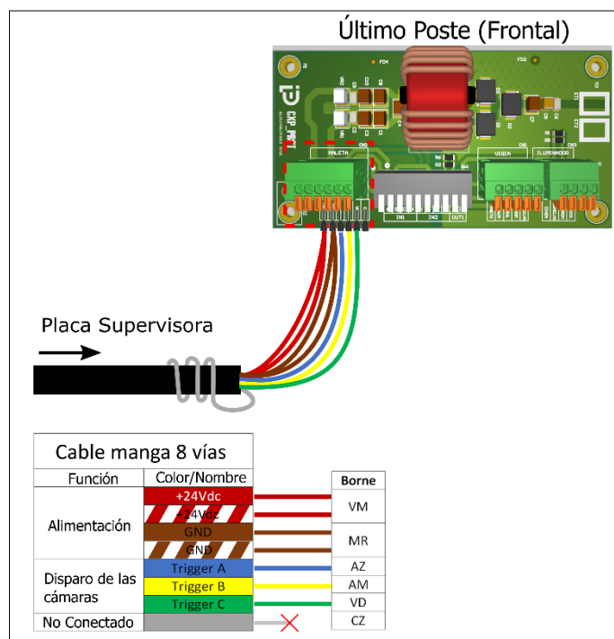
Figura 24 - Diagrama de cableado del cable de manga de 8 núcleos en la caja de conexiones del poste de captación frontal con placa de conexión 2.0
