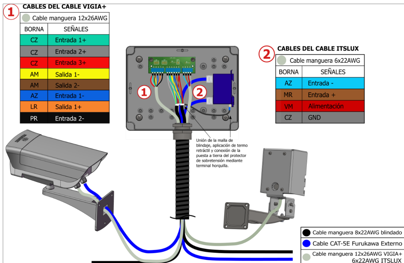
Figura 15 - Diagrama de Conexiones del dispositivo ITSCAM VIGIA+ e ITSLUX en el Poste Panorámico (con iluminador) con placa de conexión 1.0
