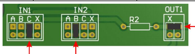
Figura 28 - Configuración de la placa de conexión 1.0 de la Caja de Paso para el dispositivo de captura de imagen Panorámica
