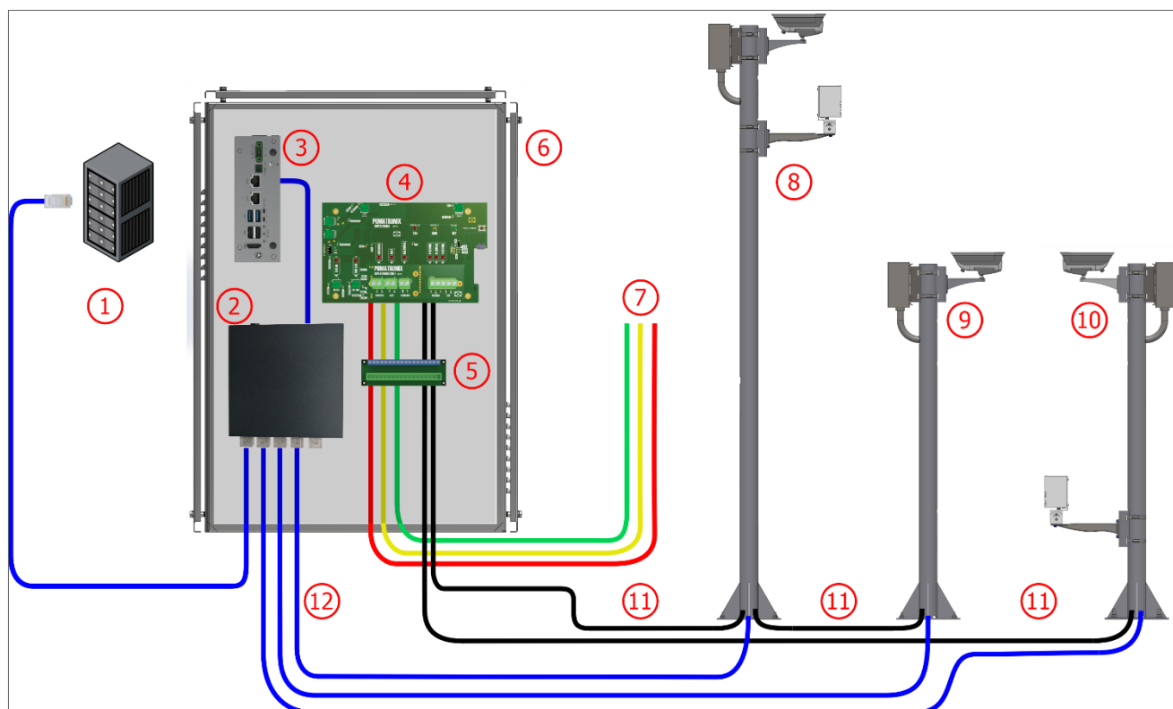
Figura 14 - Diagrama de Instalación del NEVADA en una pista: 1) Red de la concesionaria, 2) Switch, 3) ULP - Unidad Local de Procesamiento, 4) Placa Supervisora, 5) Conector General, 6) Cuadro NEVADA o Cuadro NEVADA Compacto, 7) Señales de la Pista, 8) Poste Imagen Panorámica, 9) Poste Imagen Trasera, 10) Poste Imagen Frontal, 11) Cable tipo manga 8x22AWG blindado, 12) Cable CAT-5E Furukawa Externo
