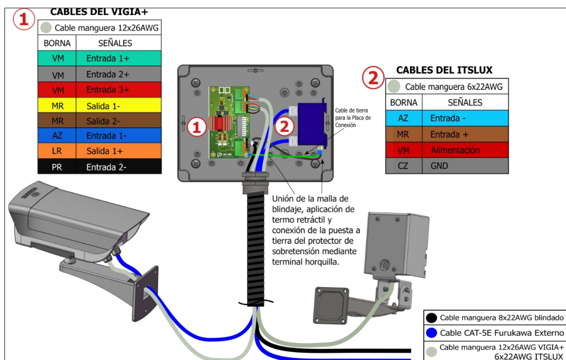
Figura 20 - Diagrama de Conexiones del dispositivo ITSCAM VIGIA+ e ITSLUX en el Poste Frontal con placa de conexión 2.0
