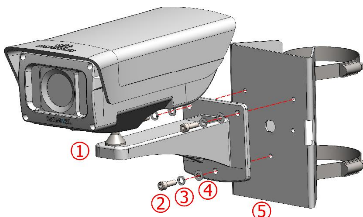
Figura 8 - Piezas del Soporte para Poste VIGIA
