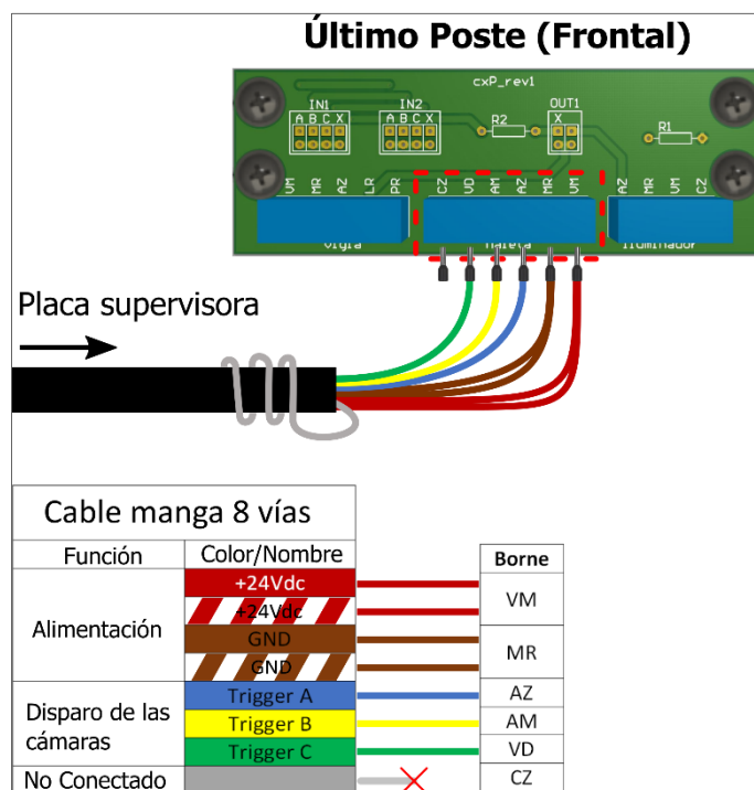
Figura 23 - Diagrama de cableado del cable de manga de 8 núcleos en la caja de conexiones del poste de captación frontal con placa de conexión 1.0
