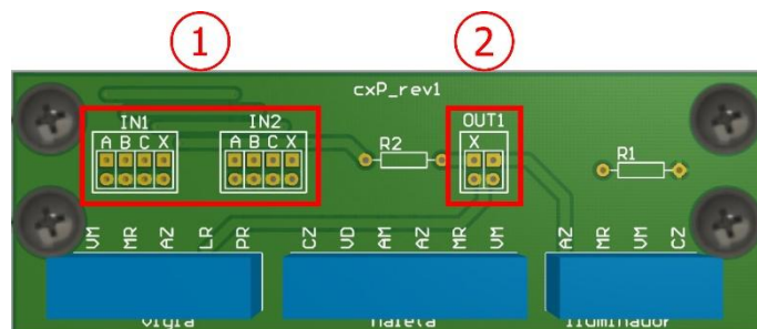
Figura 25 - Conexiones disponibles en la placa de conexión 1.0 de la Caja de Paso: 1) Señales de Entrada, 2) Señal de Salida
