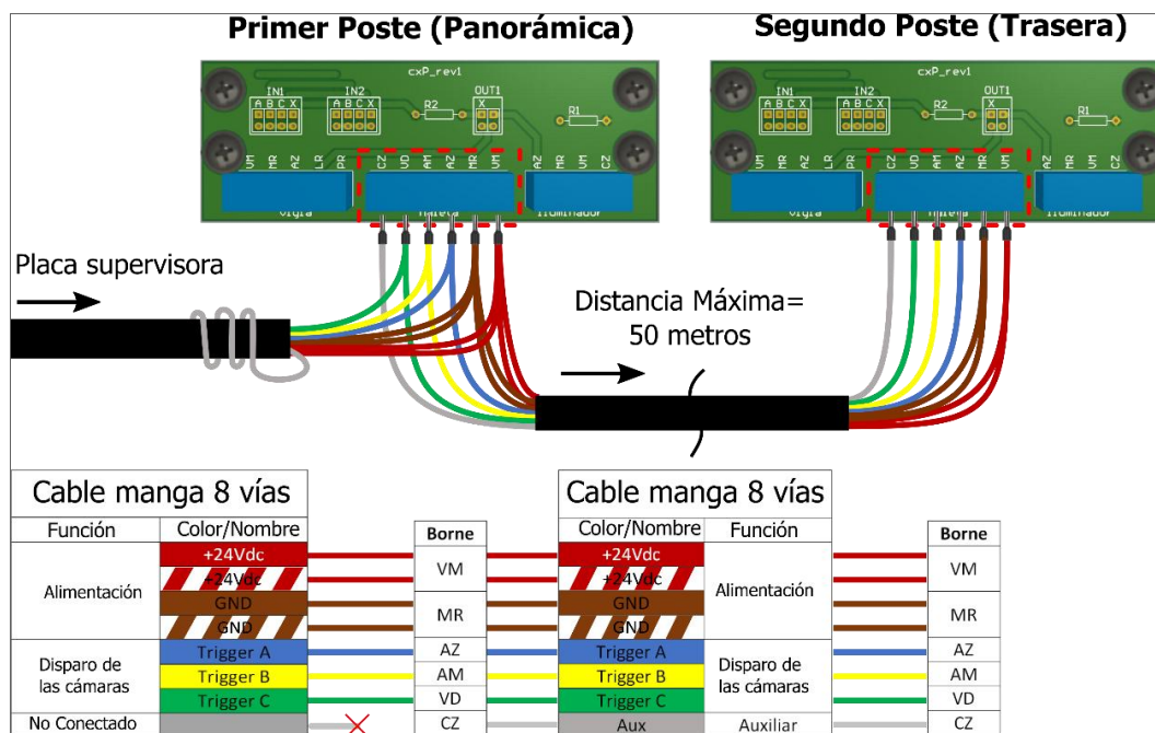
Figura 21 - Diagrama de cableado para el cable de manguito de 8 vías en cada caja de conexiones de los postes de captura panorámicos y traseros con placa de conexión 1.0
