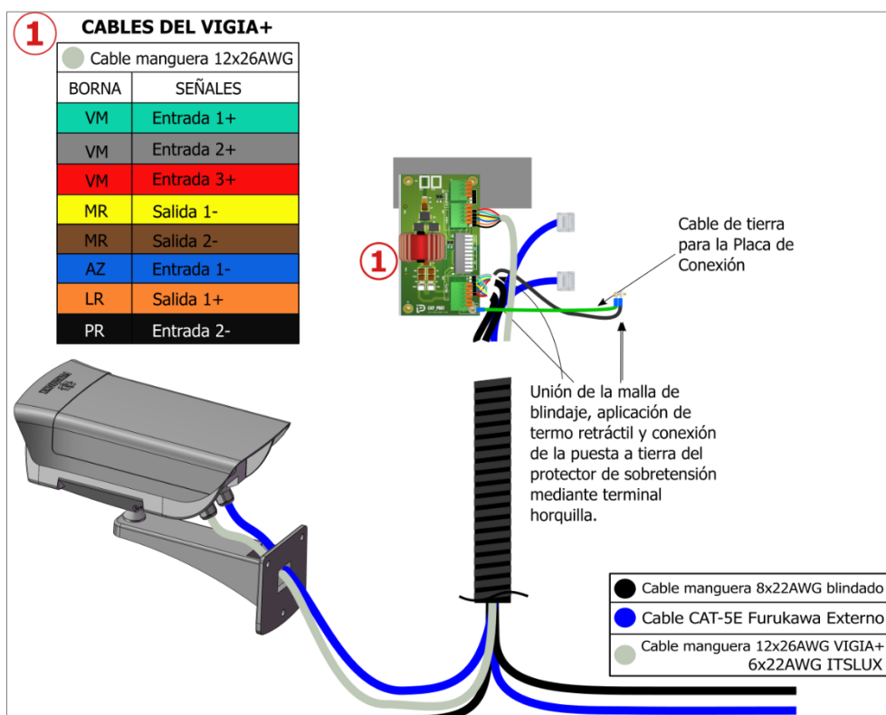
Figura 18 - Diagrama de Conexiones del dispositivo ITSCAM VIGIA+ en el Poste Trasero o Panorámico (sin iluminador) con placa de conexión 2.0
