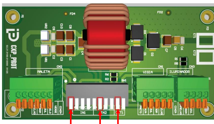
Figura 31 - Configuración de la placa de conexión 2.0 de la Caja de Paso para el dispositivo de captura de imagen Trasera
