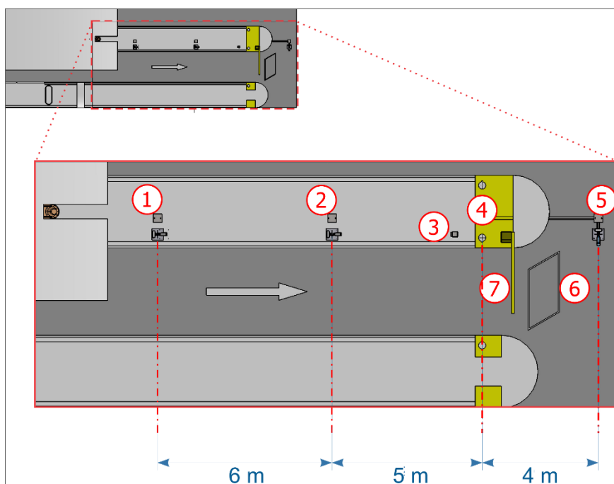
Figura 1 - Vista superior de la instalación en una pista de cobro automático (AVI): 1) Poste de captura Panorámica, 2) Poste de captura Trasera, 3) Semáforo de la pista, 4) Barrera Óptica de la pista, 5) Poste de captura Frontal, 6) Lazo de la pista, 7) Barrera de la pista
