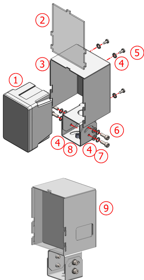
Figura 9 - Piezas del Soporte ITSLUX NEVADA
