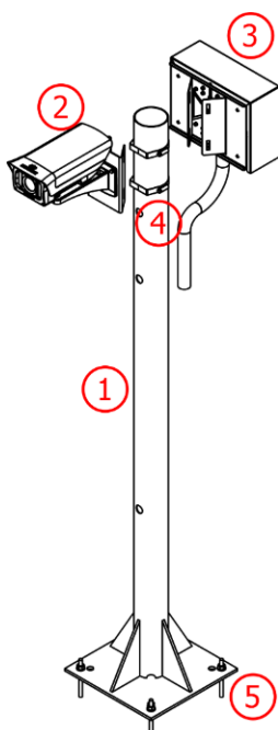
Figura 12 - Poste de Captura de imagen Trasera
