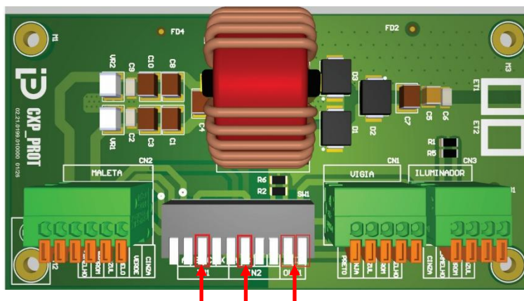
Figura 32 - Configuración de la placa de conexión 2.0 de la Caja de Paso para el dispositivo de captura de imagen Panorámica
