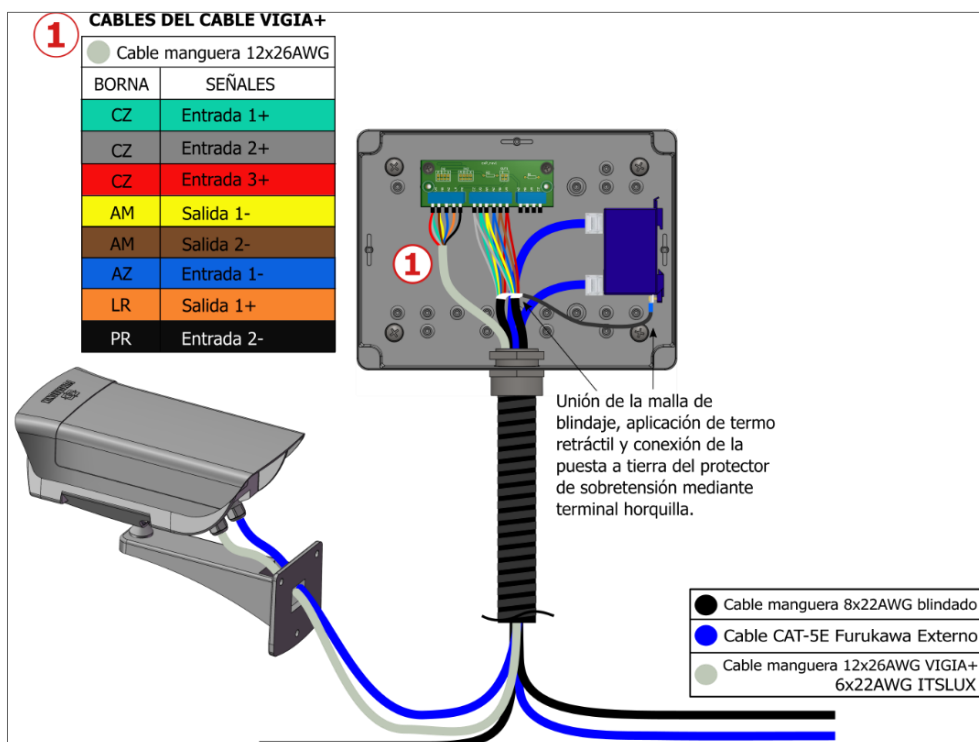
Figura 17 - Diagrama de Conexiones del dispositivo ITSCAM VIGIA+ en el Poste Trasero o Panorámico (sin iluminador) con placa de conexión 1.0
