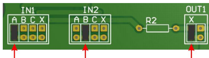
Figura 27 - Configuración de la placa de conexión 1.0 de la Caja de Paso para el dispositivo de captura de imagen Trasera
