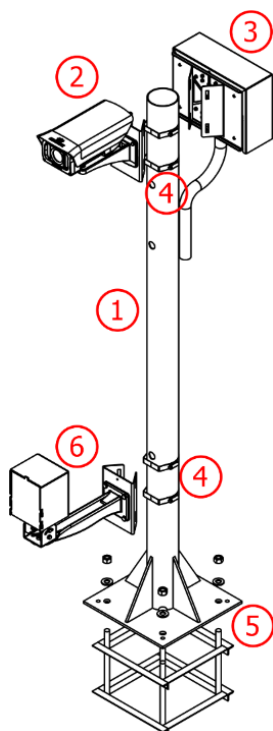
Figura 13 - Poste de Captura de imagen Frontal
