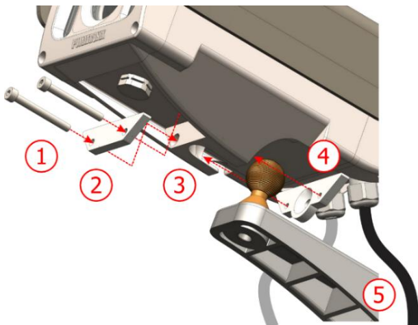
Figura 7 - Piezas del Soporte VIGIA+
