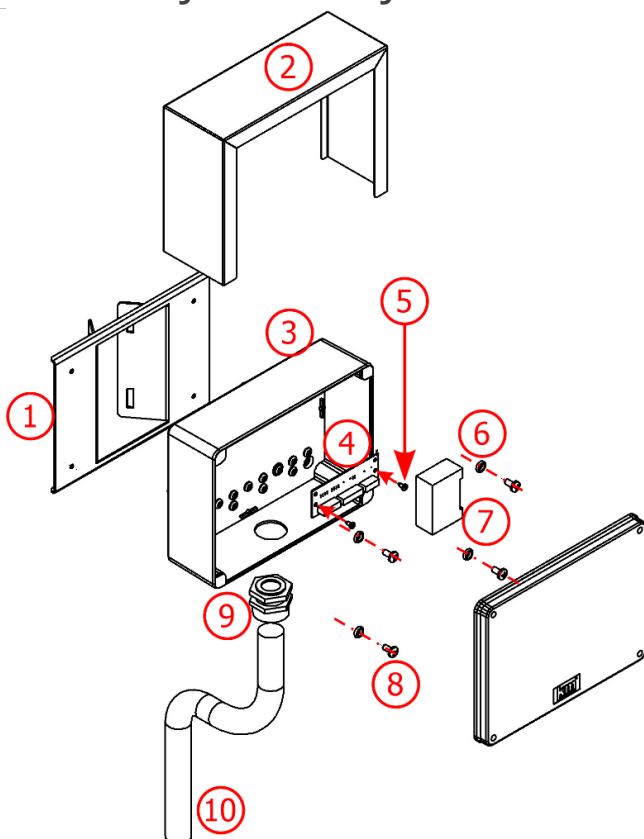
Figura 6 - Componentes de la Caja de Paso
