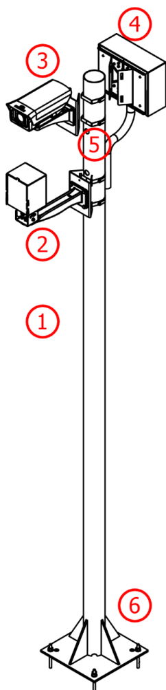
Figura 11 - Poste de Captura de imagen Panorámica
