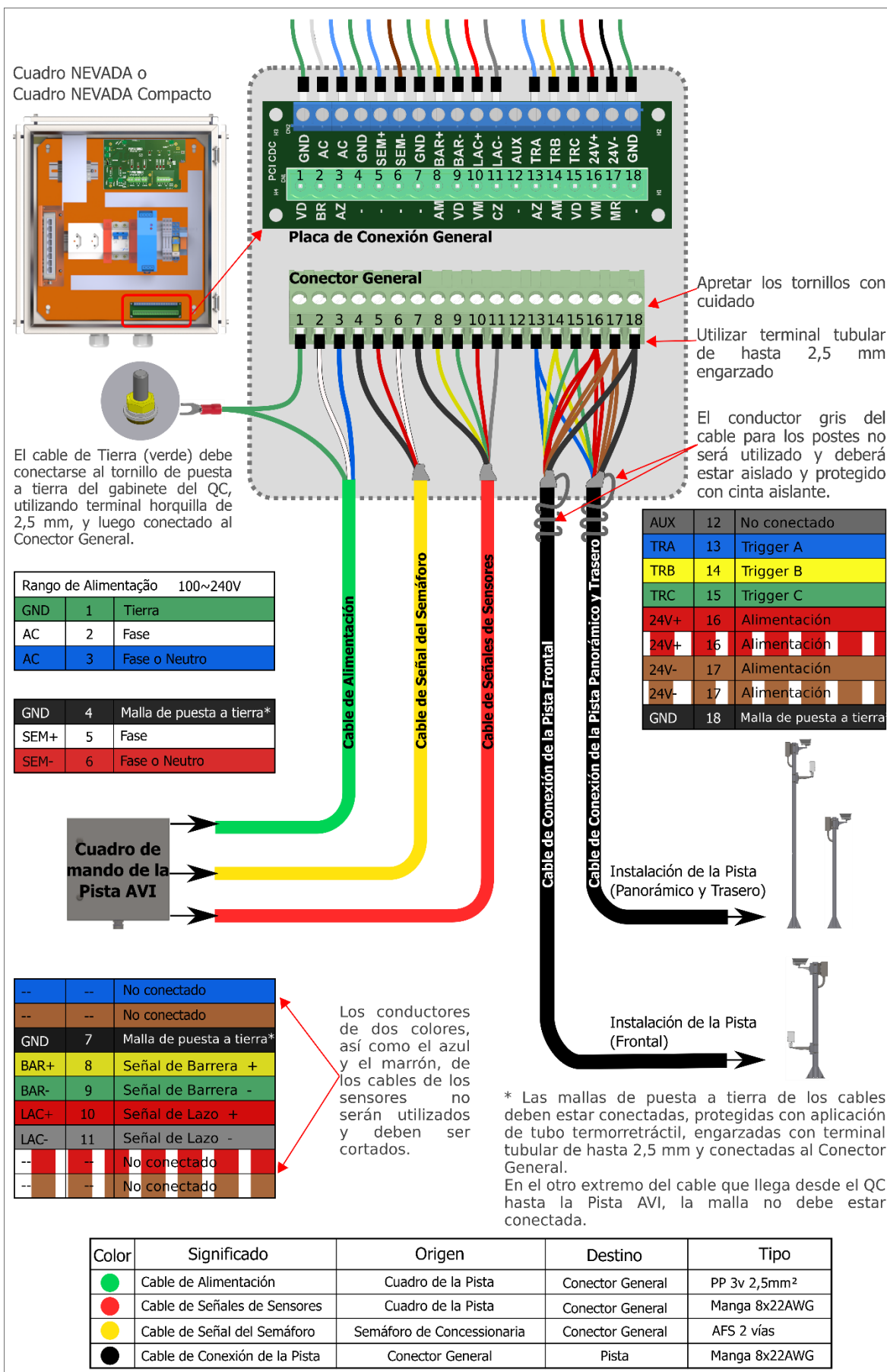
Figura 33 - Esquema de Conexiones con la Placa de Conexión General (2 cables para pista)
