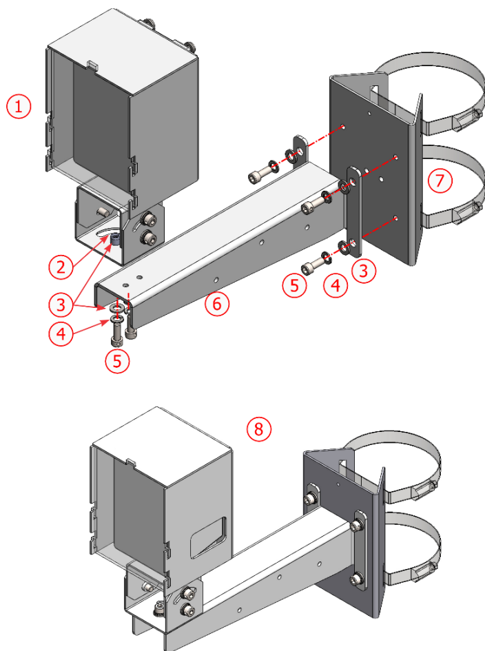
Figura 10 - Piezas para fijación del Soporte ITSLUX NEVADA al Soporte para Poste
