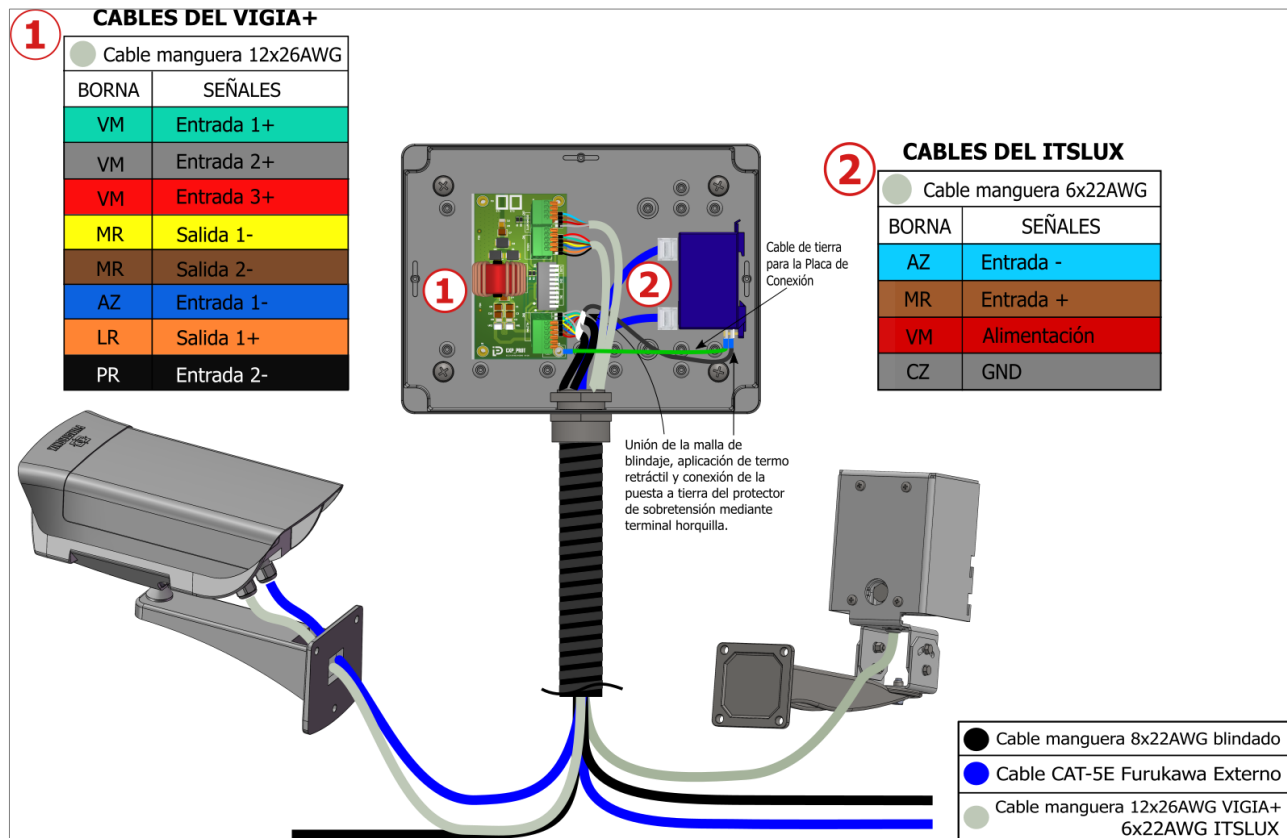
Figura 16 - Diagrama de Conexiones del dispositivo ITSCAM VIGIA+ e ITSLUX en el Poste Panorámico (con iluminador) con placa de conexión 2.0
