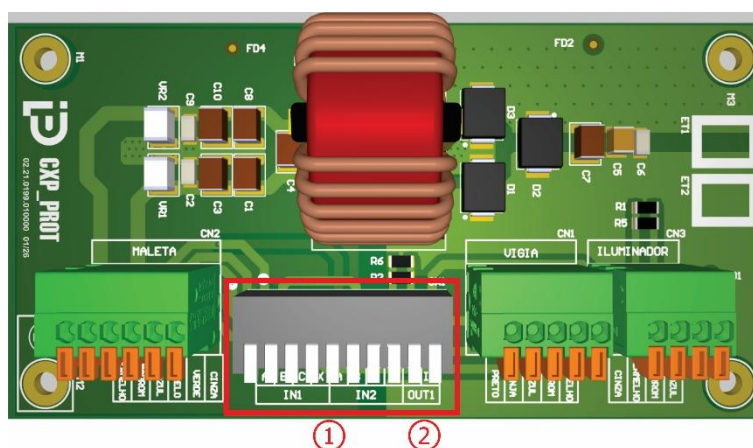
Figura 29 - Conexiones disponibles en la placa de conexión 2.0 de la Caja de Paso: 1) Señales de Entrada, 2) Señal de Salida
