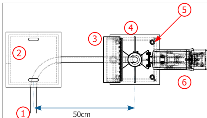
Figura 5 - Posicionamiento del poste de captura Frontal en asfalto: 1) Tubería de protección de cables, 2) Caja de Inspección con tapa de hierro fundido, 3) Caja de Paso fijada al poste, 4) Base del poste, 5) Punto de fijación al anclaje de 190 mm, 6) ITSCAM VIGIA+ fijada al poste
