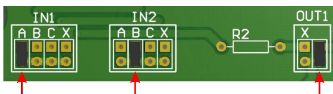
Figura 26 – Ejemplo de configuración de la placa de conexión 1.0 de la Caja de Paso para el dispositivo de captura de imagen Frontal
