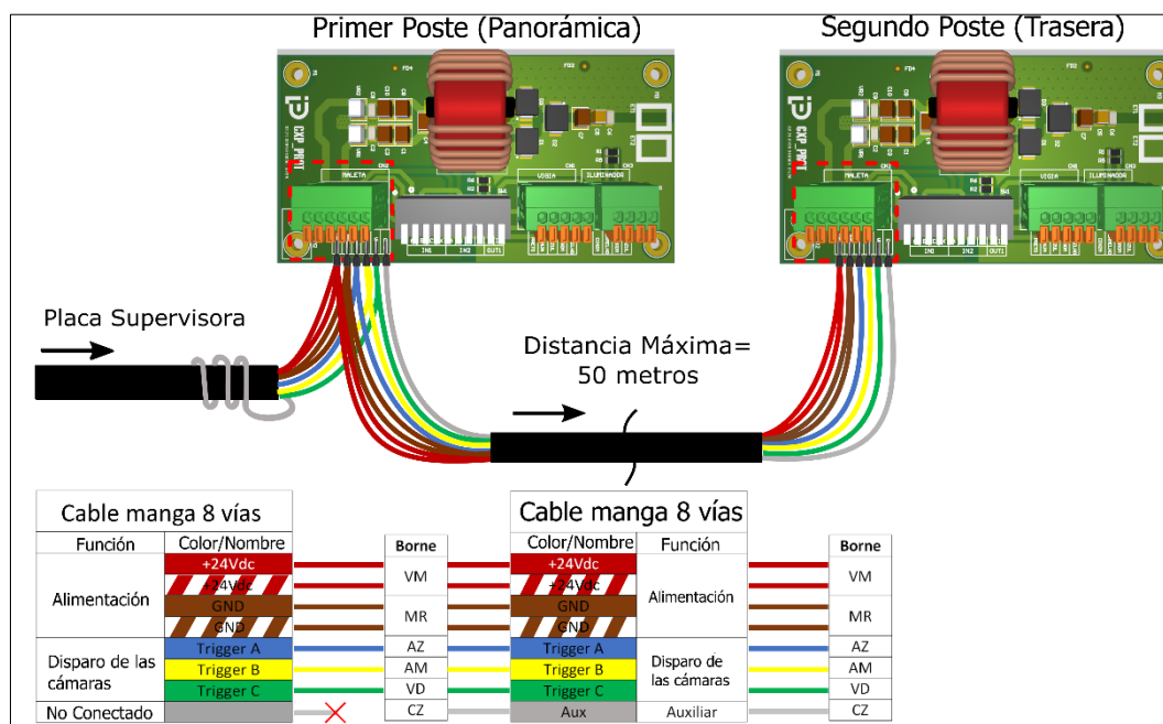
Figura 22 - Diagrama de cableado para el cable de manguito de 8 vías en cada caja de conexiones de los postes de captura panorámicos y traseros con placa de conexión 2.0
