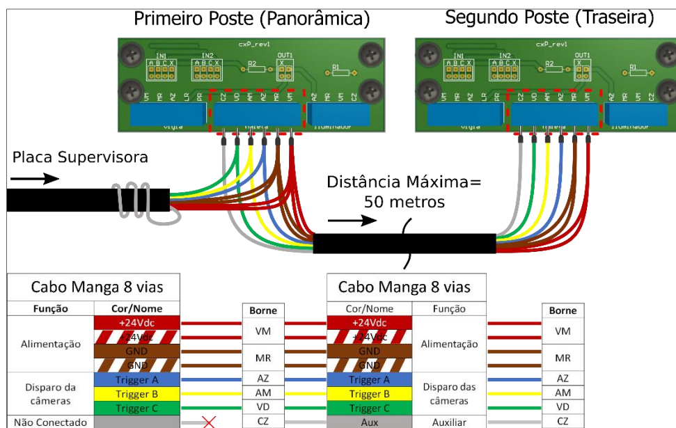
Figura 18 - Diagrama de Ligações do cabo manga 8 vias em cada Caixa de Passagem dos Postes de captura Panorâmica e captura Traseira
