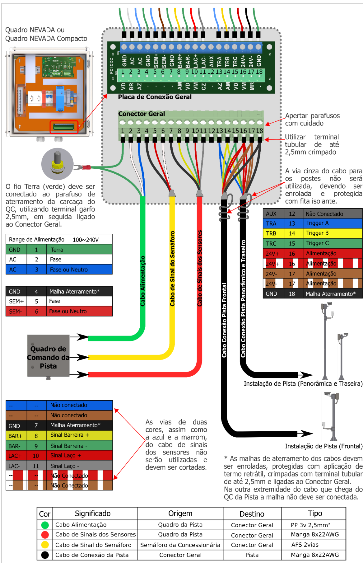
Figura 24 - Esquema de Conexões com a Placa de Conexão Geral (2 cabos para pista)
