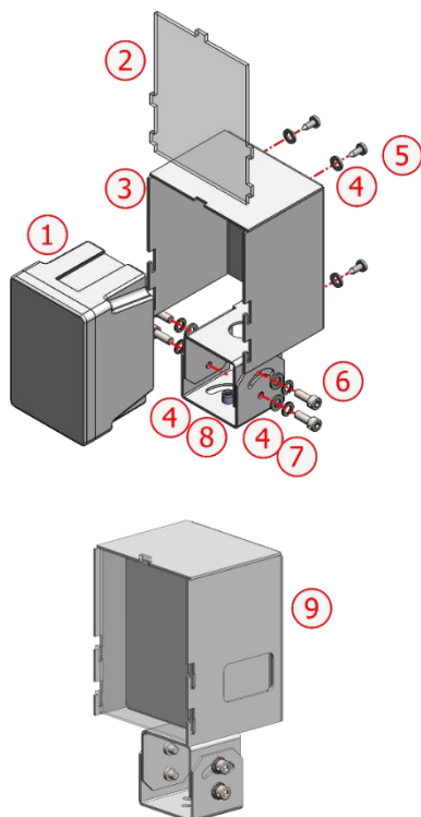
Figura 9 - Peças do Suporte ITS LUX NEVADA
