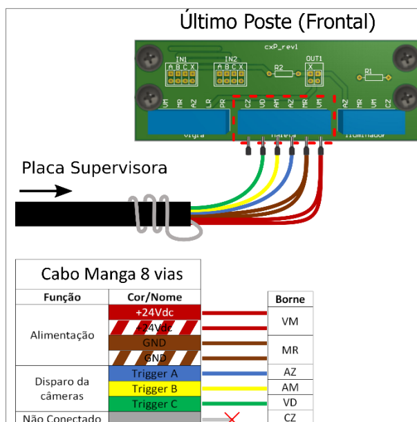
Figura 19 - Diagrama de Ligações do cabo manga 8 vias na Caixa de Passagem do Poste de captura Frontal
