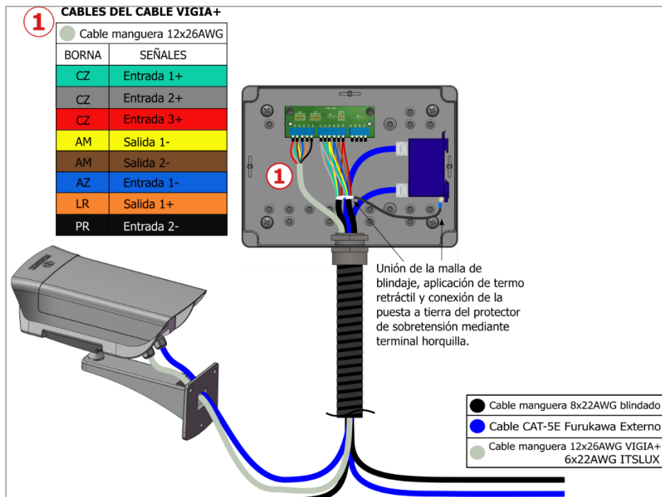
Figura 16 - Diagrama de Conexiones del dispositivo ITSCAM VIGIA+ en el Poste Trasero o Panorámico (sin iluminador)
