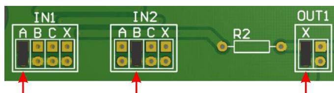
Figura 22 - Configuración de la placa de la Caja de Paso para el dispositivo de captura de imagen Trasera
