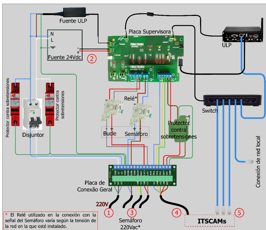
Figura 25 - Diagrama de Conexiones del Cuadro NEVADA
