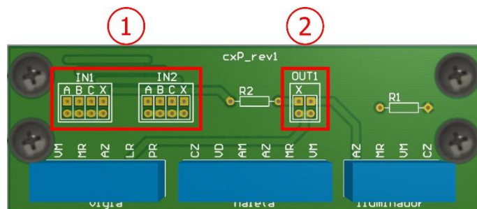
Figura 20 - Conexiones disponibles en la placa de la Caja de Paso: 1) Señales de Entrada, 2) Señal de Salida
