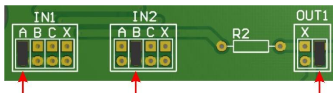
Figura 21 – Ejemplo de configuración de la placa de la Caja de Paso para el dispositivo de captura de imagen Frontal
