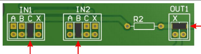
Figura 23 - Configuración de la placa de la Caja de Paso para el dispositivo de captura de imagen Panorámica
