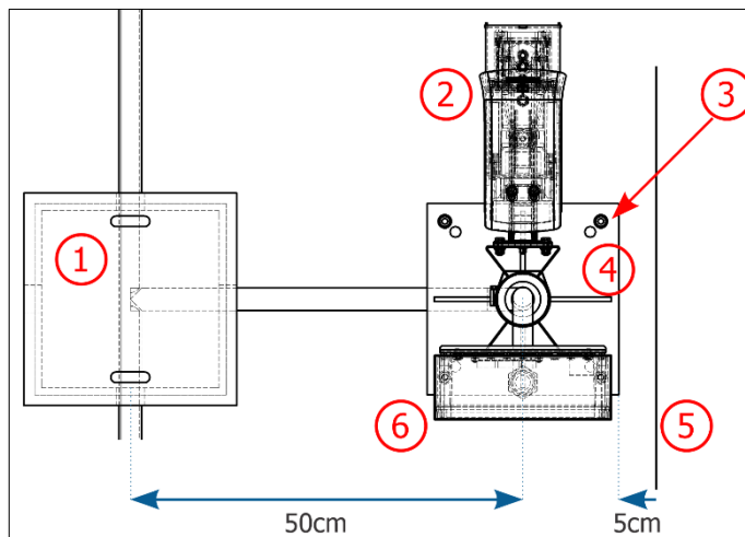
Figura 3 - Posicionamiento del poste de captura Panorámica o Trasera: 1) Caja de Inspección con tapa de hierro fundido, 2) ITSCAM VIGIA+ fijada al poste, 3) Anclajes tipo Parabolt, 4) Base del poste, 5) Borde de la acera existente, 6) Caja de Paso fijada al poste
