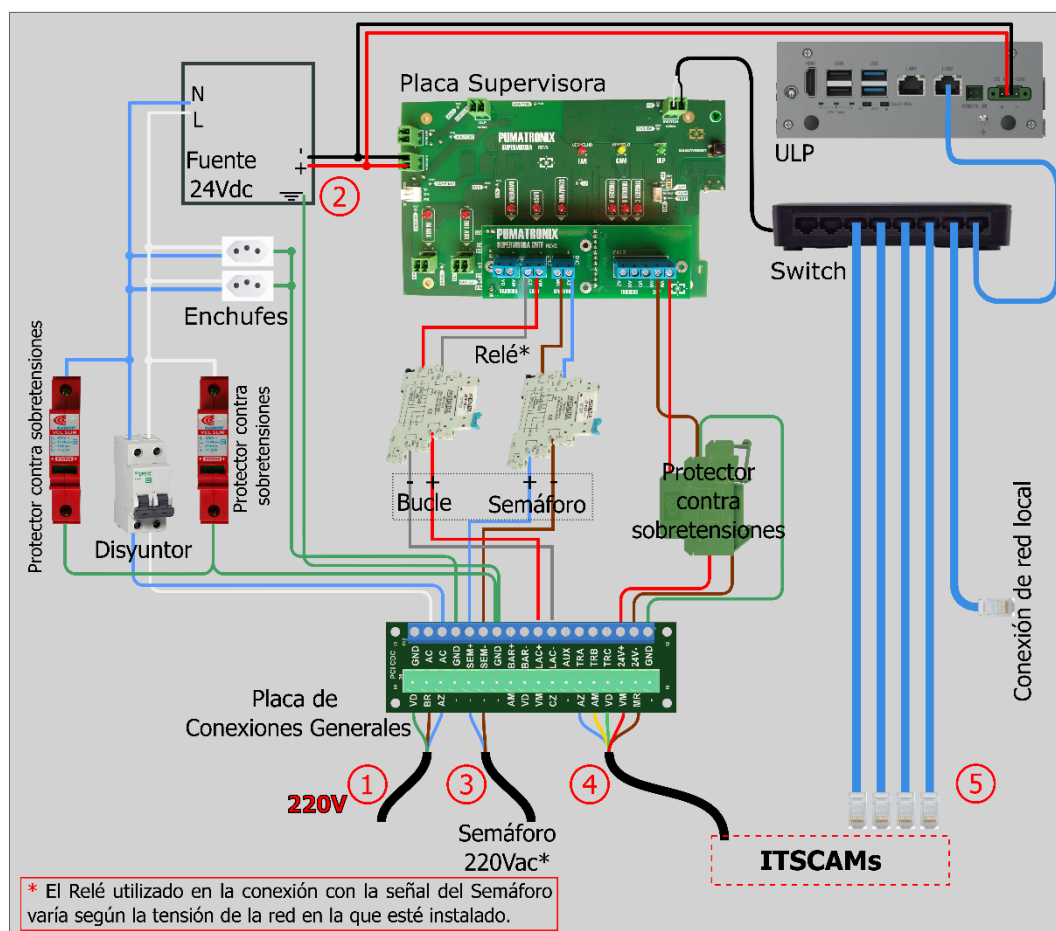
Figura 26 - Diagrama de Conexiones del Cuadro NEVADA Compacto
