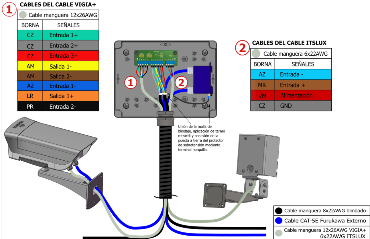
Figura 15 - Diagrama de Conexiones del dispositivo ITSCAM VIGIA+ e ITSLUX en el Poste Panorámico (con iluminador)
