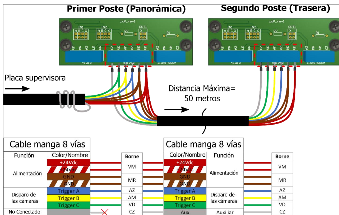
Figura 18 - Diagrama de cableado para el cable de manguito de 8 vías en cada caja de conexiones de los postes de captura panorámicos y traseros
