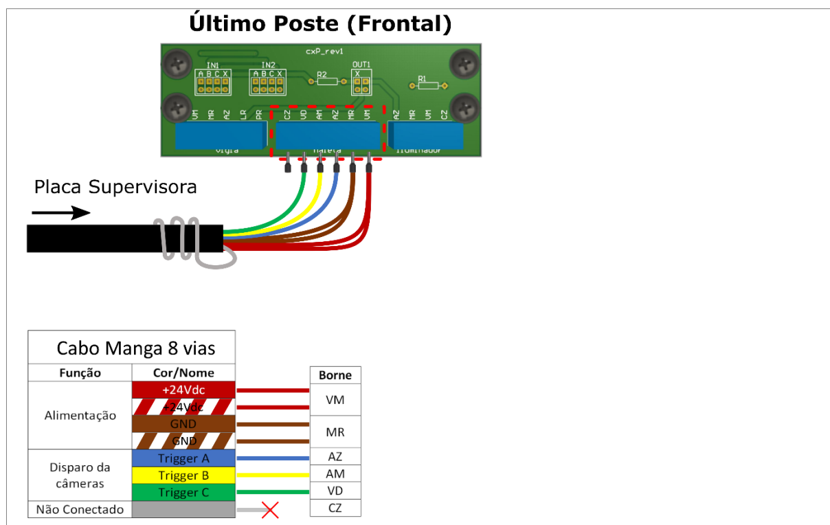
Figura 19 - Diagrama de Ligações do cabo manga 8 vias na Caixa de Passagem do Postes de captura Frontal
