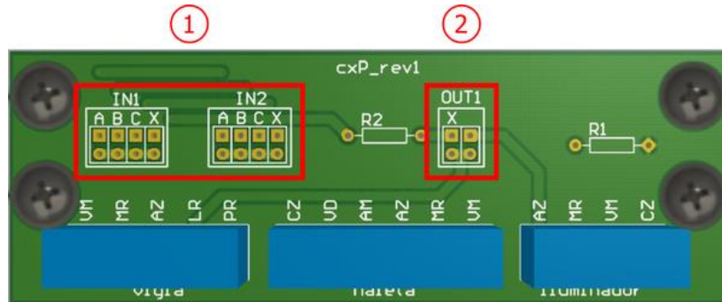
Figura 20 - Conexões disponíveis na placa da Caixa de Passagem: 1) Sinais de Entrada, 2) Sinal de Saída
