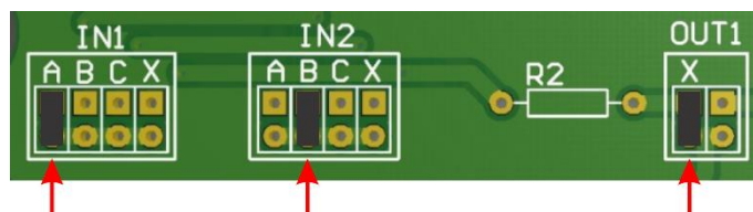
Figura 22 - Configuração da placa da Caixa de Passagem para o dispositivo de captura de imagem Traseira
