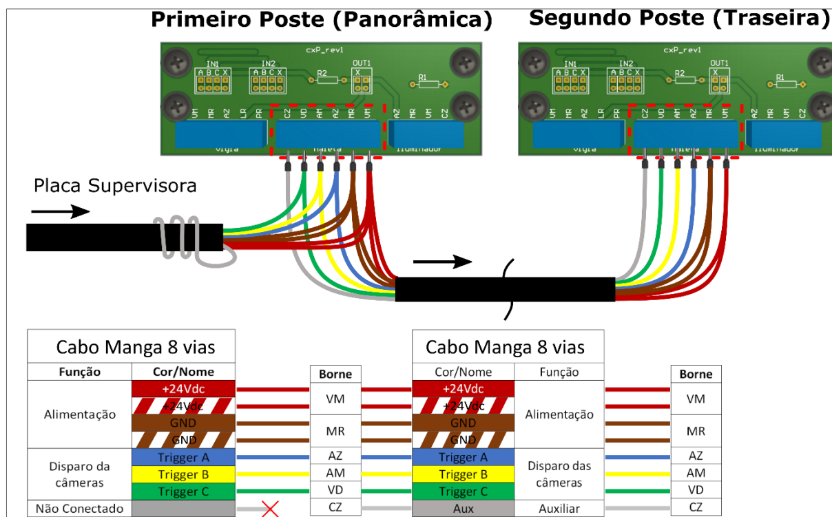
Figura 18 - Diagrama de Ligações do cabo manga 8 vias em cada Caixa de Passagem dos Postes de captura Panorâmica e captura Traseira
