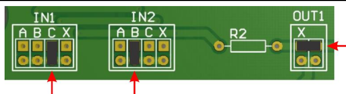
Figura 23 - Configuração da placa da Caixa de Passagem para o dispositivo de captura de imagem Panorâmica
