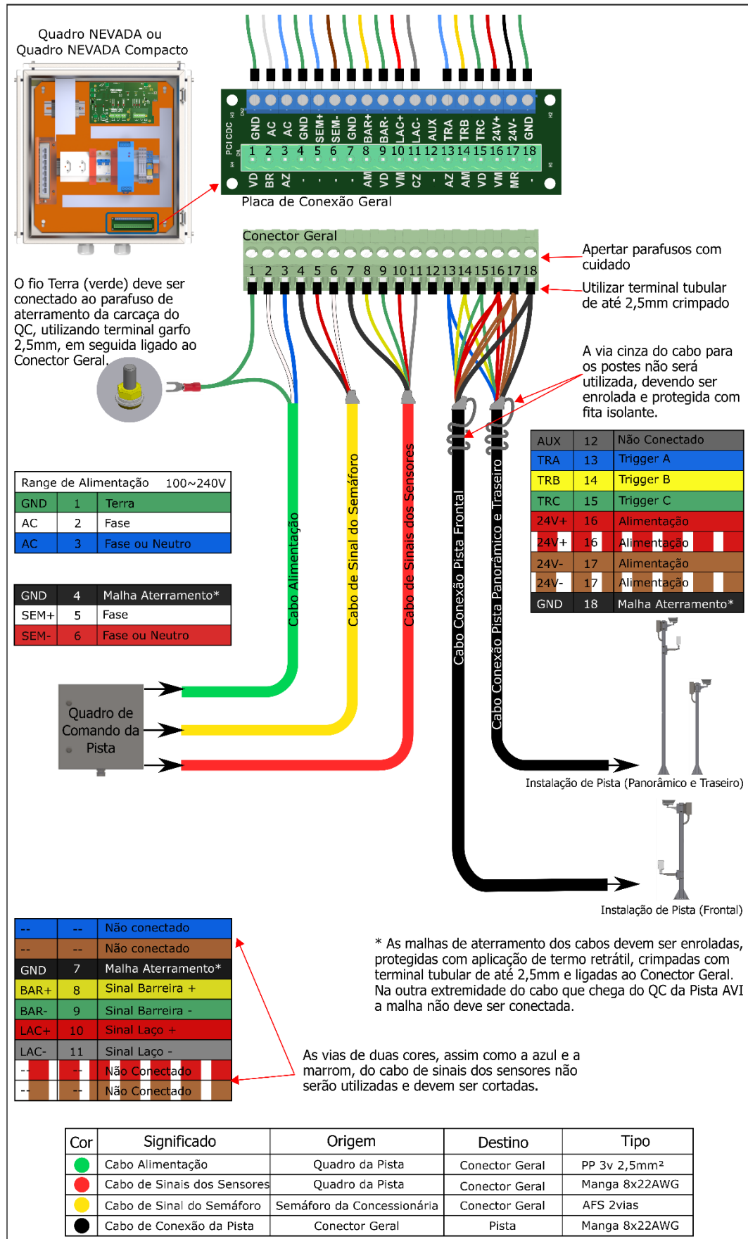
Figura 24 - Esquema de Conexões com a Placa de Conexão Geral
