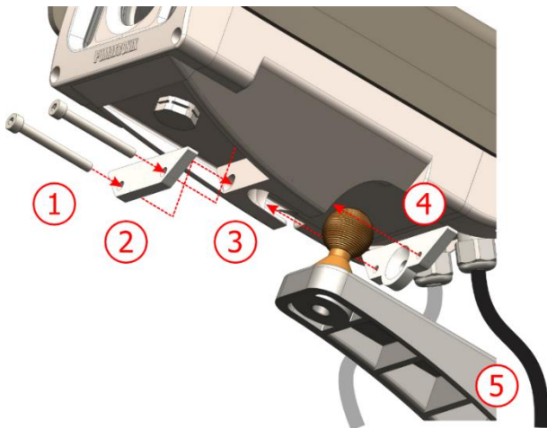
Figura 7 - Piezas del Soporte VIGÍA+
