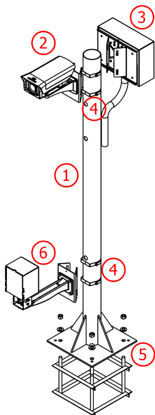
Figura 12 - Poste de captura de imagen Delantera
