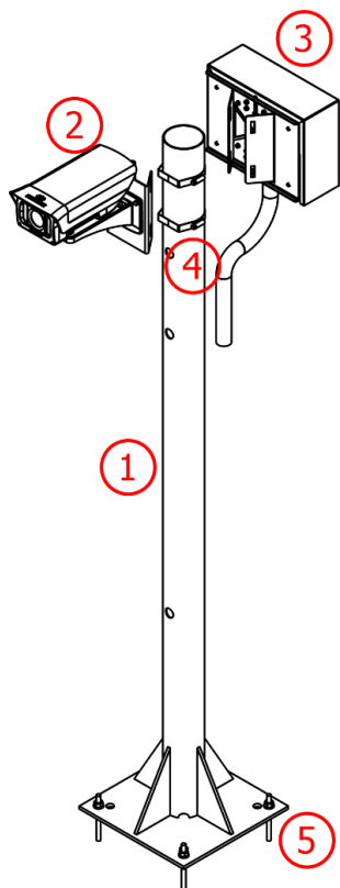
Figura 13 - Poste de captura de imagen Trasera
