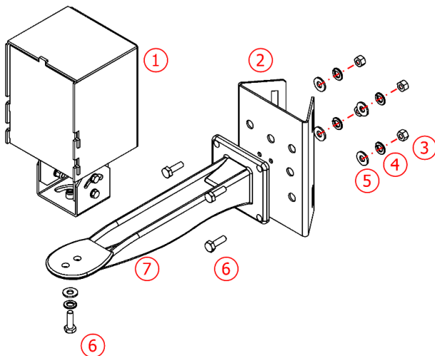
Figura 10 - Piezas del Soporte Celda del resaltador ITSLUX
