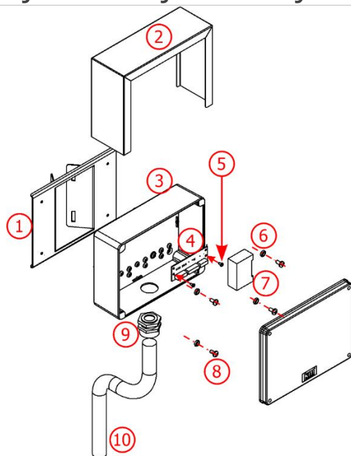
Figura 6 - Componentes de la Caja de Pasaje
