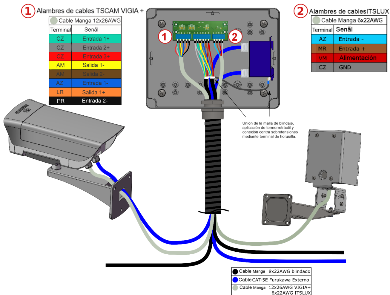
Figura 17 - Conexión del dispositivo ITSCAM VIGIA+ e ITSLUX al Poste Frontal
