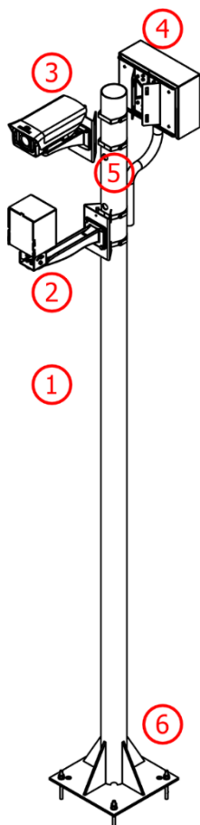
Figura 11 - Poste de captura de imagen Panorámica
