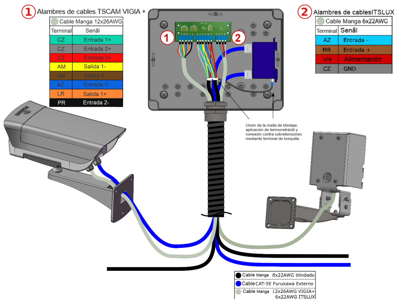
Figura 15 - Conexiones del dispositivo ITSCAM VIGÍA+ e ITSLUX en el Poste Panorámico (con iluminador)
