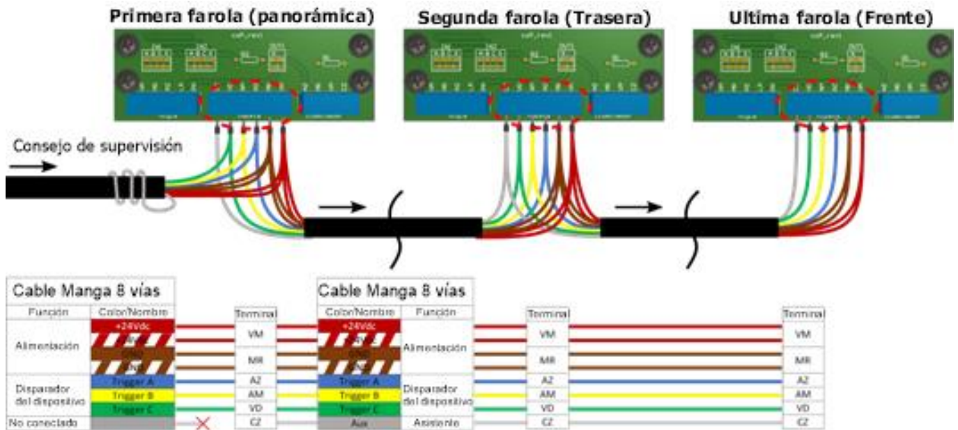
Figura 18 - Conexiones de cables manguitos de 8 vías en las cajas de conexiones de los respectivos postes
