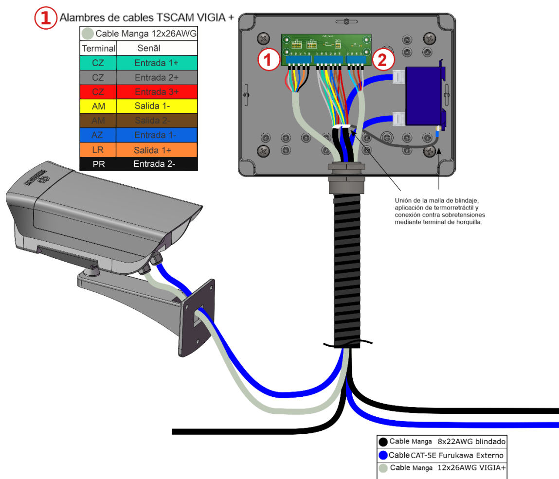
Figura 16 - Conexión del dispositivo ITSCAM VIGIA+ al Poste Trasero o Panorámico (sin iluminador)
