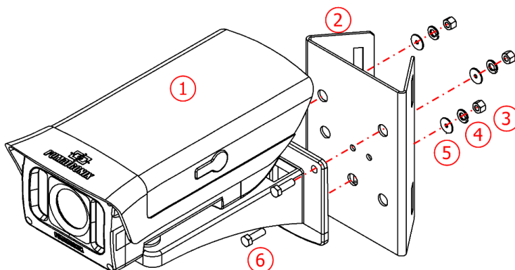
Figura 8 - Piezas de soporte de celda del dispositivo ITSCAM VIGÍA+
