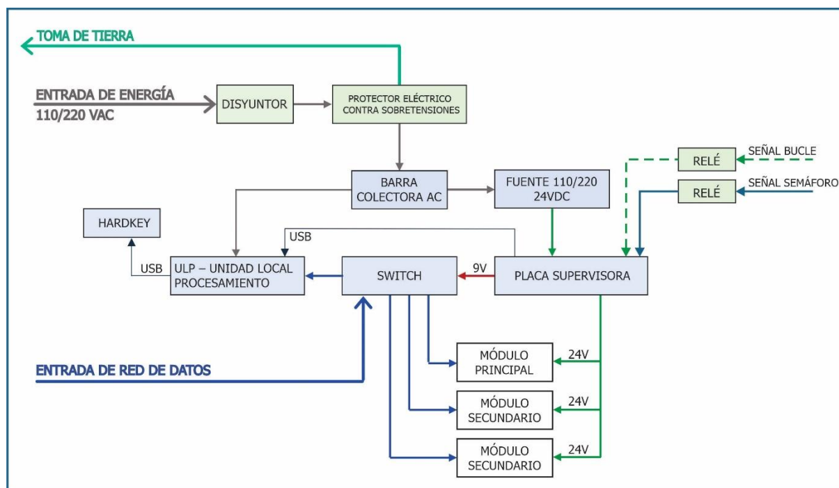
Figura 9 - Diagrama de instalación del cuadro NM1 compacto
