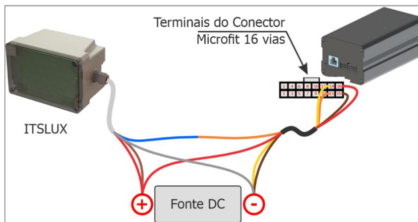
Figura 16 - Diagrama ilustrativo de las conexiones del dispositivo ITSCAM con el iluminador ITSLUX
