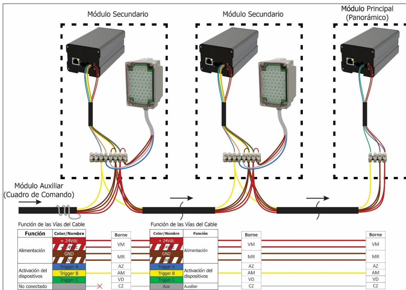
Figura 13 – Diagrama de conexiones entre módulos
