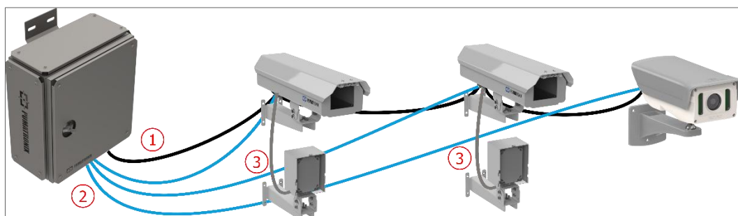
Figura 3 – Diagrama general de la instalación de cables y dispositivos: 1) Cable de manga de 8 vías; 2) Cables Ethernet; 3) Cable ITSLUX
