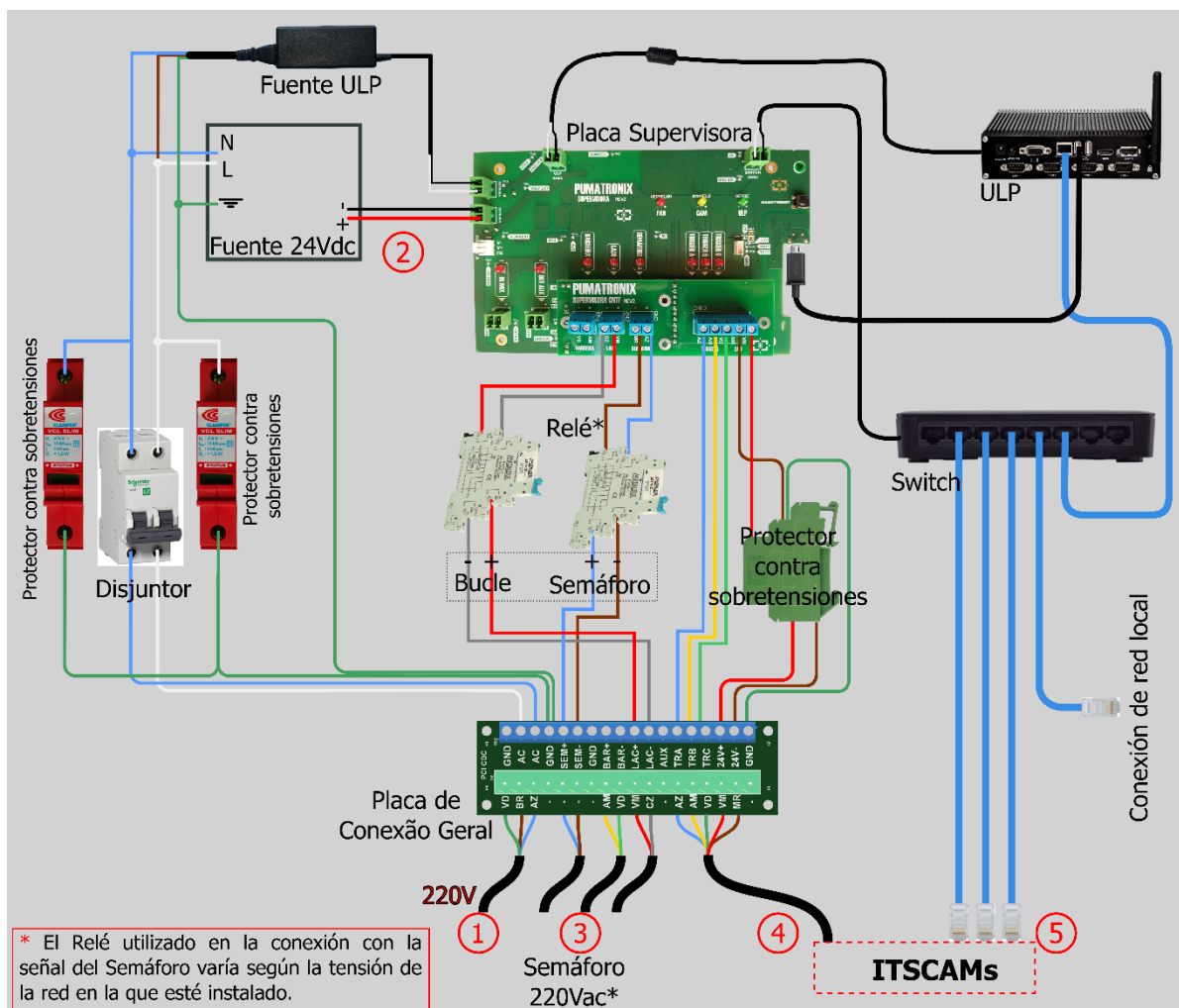
Figura 11 - Diagrama de conexiones con la Placa Supervisora (cuando Semáforo 220 Vca)
