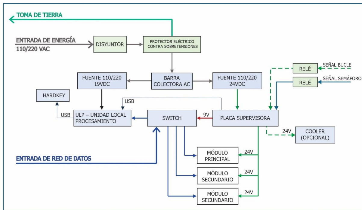
Figura 8 - Diagrama de instalación del cuadro NM1
