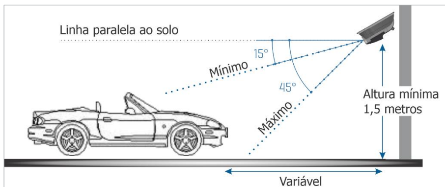
Figura 18 - Vista Lateral da instalação Posicionamento Frontal
