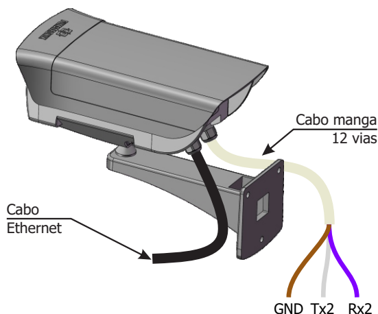
GND Tx2 Rx2
